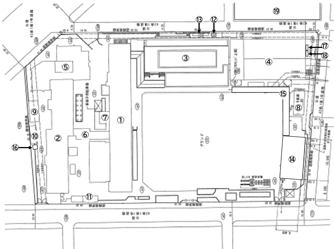
配置図
