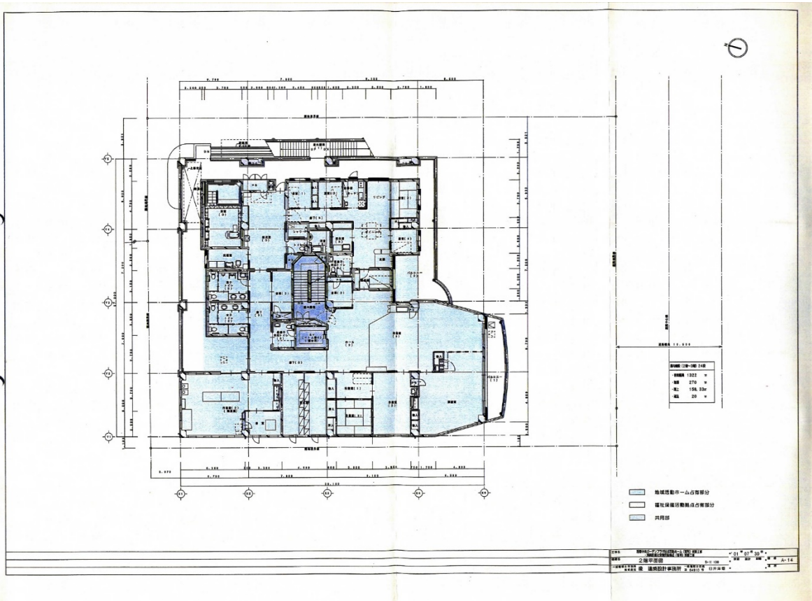
< 3 階平面図 >
