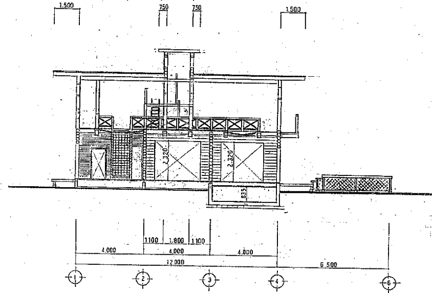
断面図 S: 1/100
