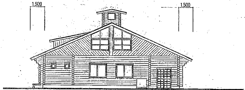
北側立面図
