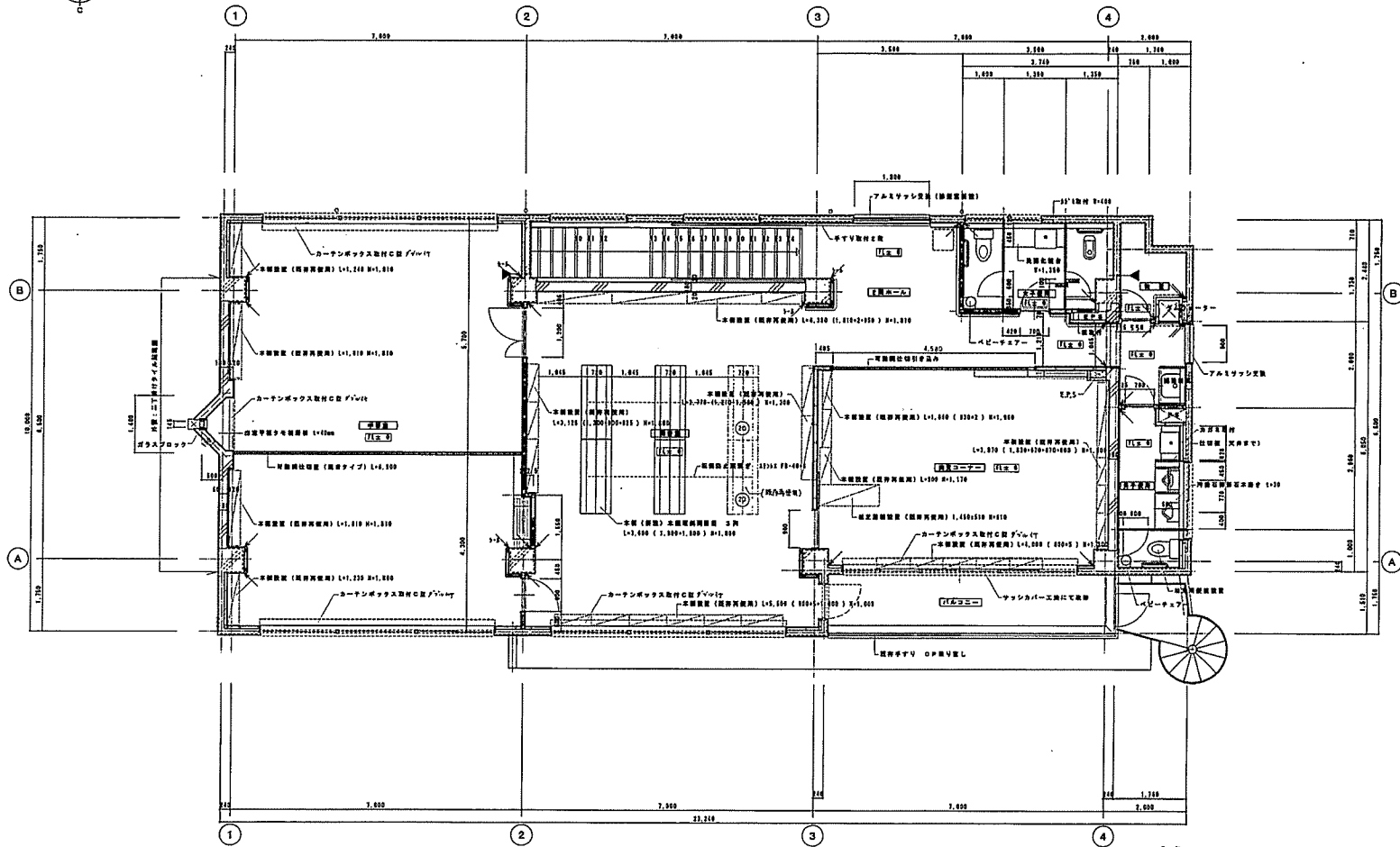
改修後 2階平面図 1/110
