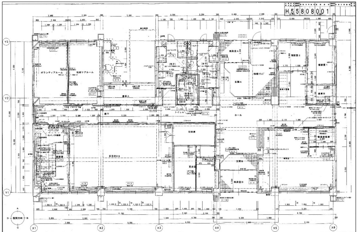
1階（平面詳細図）
