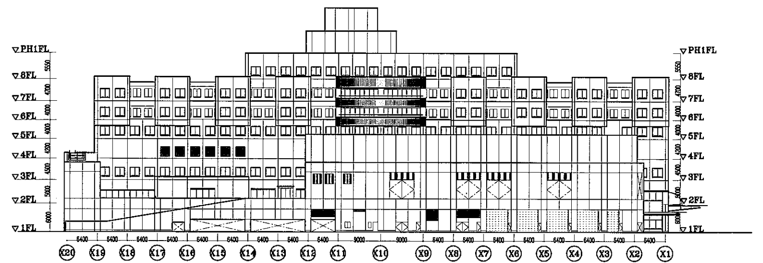
北面立面図 S=1/800
