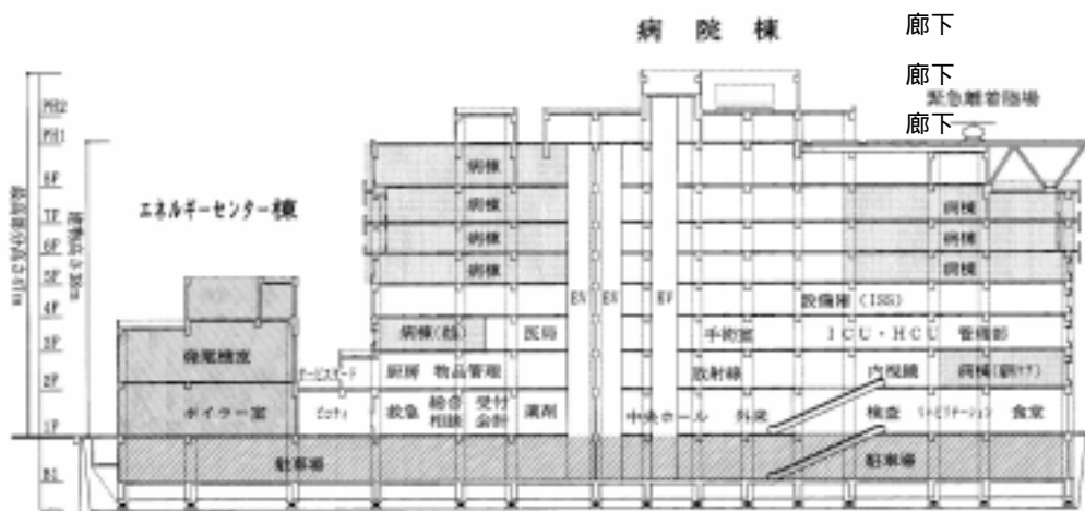
病院正面方向から見た断面
