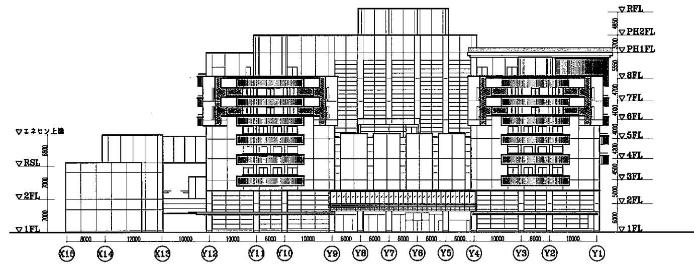
西面立面図 S=1/800
