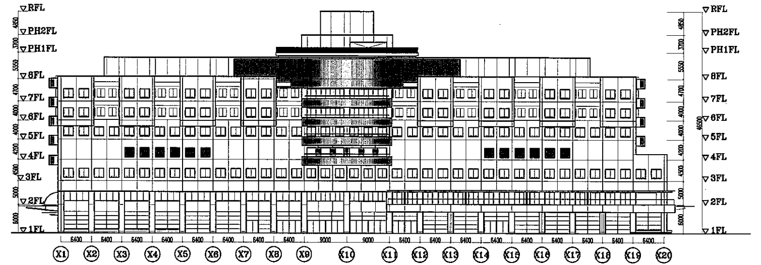
南面立面図 S=1/800
