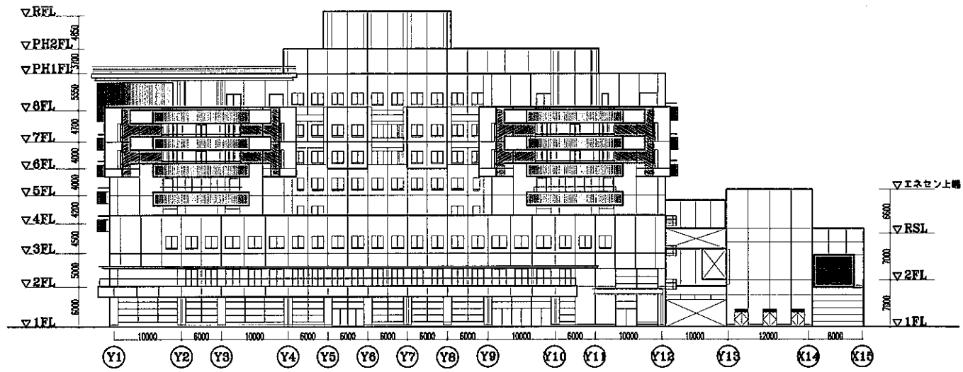
東面立面図 S=1/800
