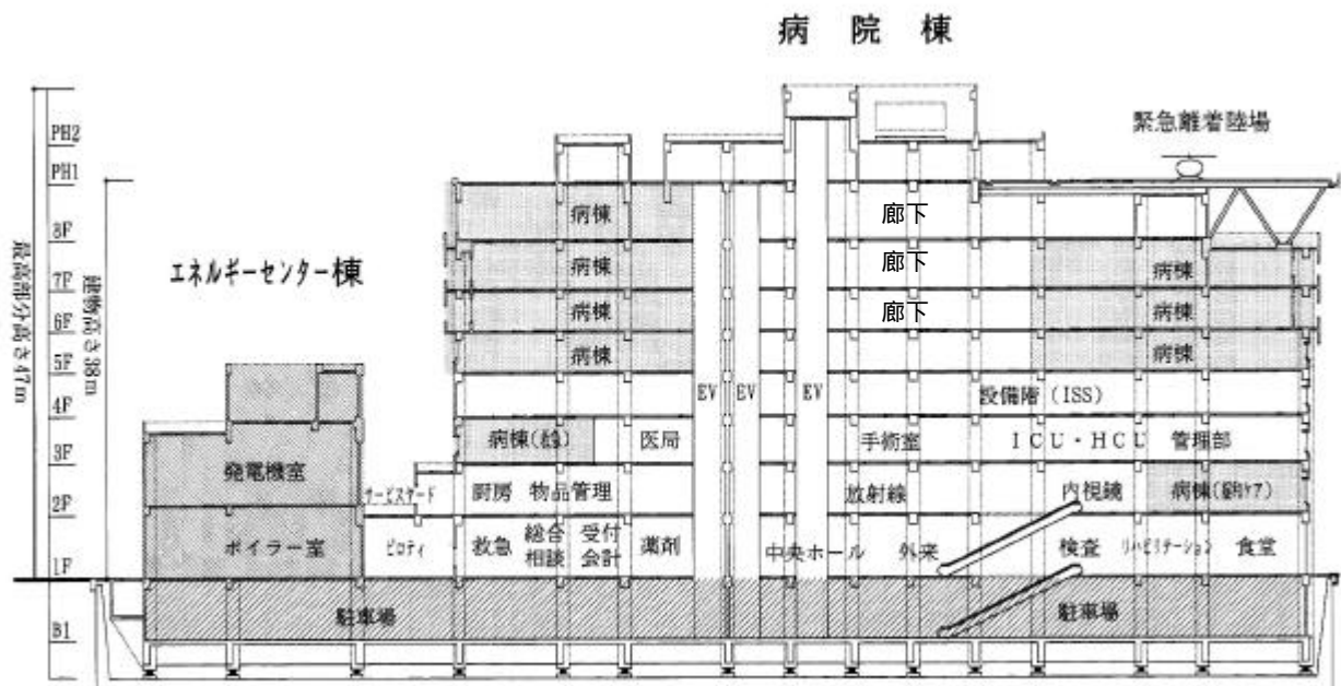
病院正面方向から見た断面
