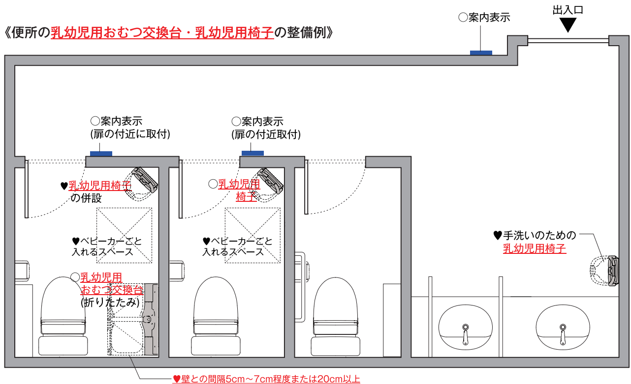
図20-4 乳幼児連れ利用者に配慮した便所の整備例
