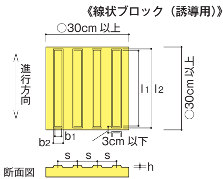
図16-1 線状ブロック等・点状ブロック等の構造
