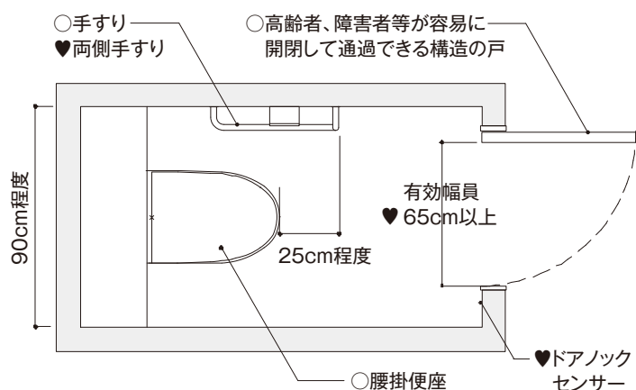
図9-9 その他の便房の例
