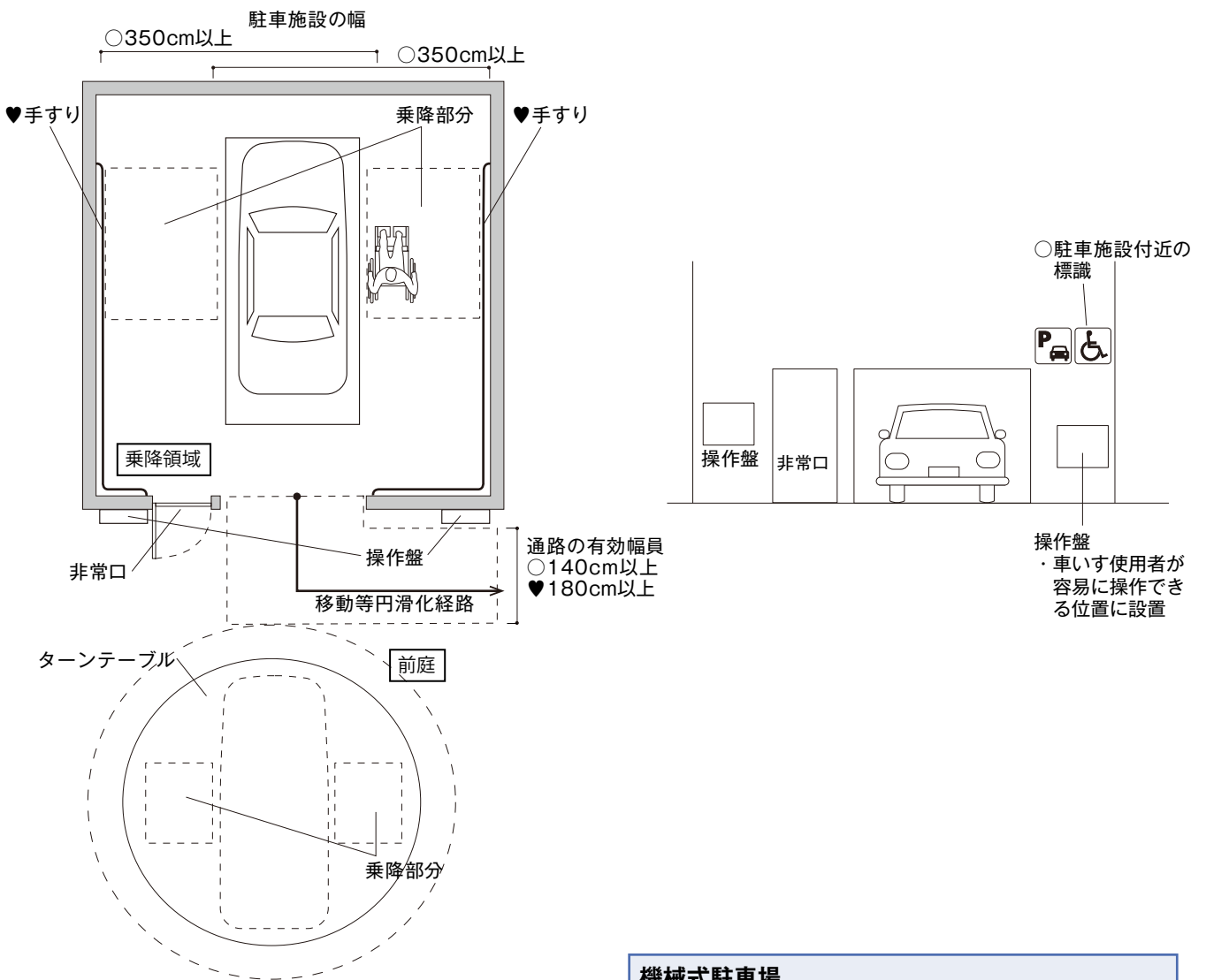
図3-2 機械式駐車場の整備例
