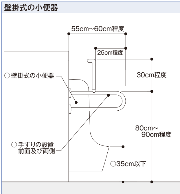
図9-8 男子用小便器の例
