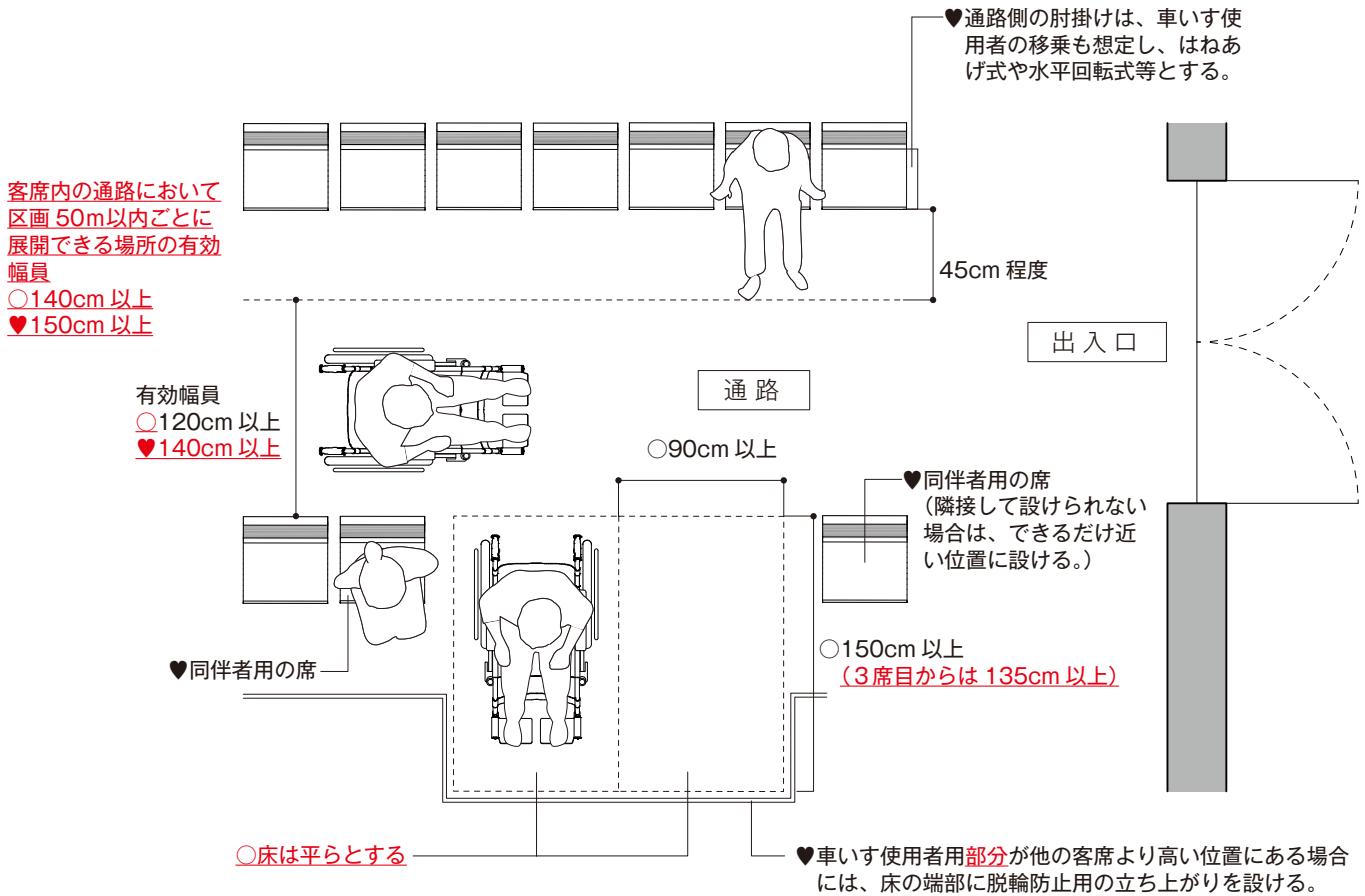
図12-2 車いす使用者用部分まわりの整備例
