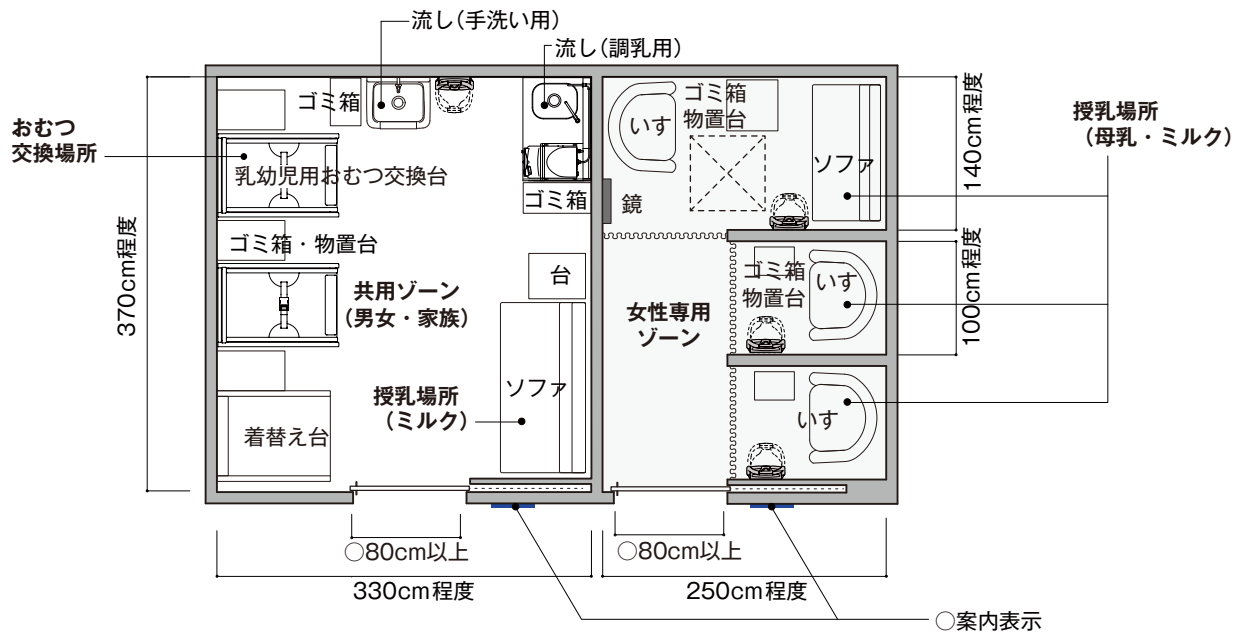
図20-2 授乳室・おむつ交換場所の整備例(共用ゾーン・母乳ゾーン入口別型)
