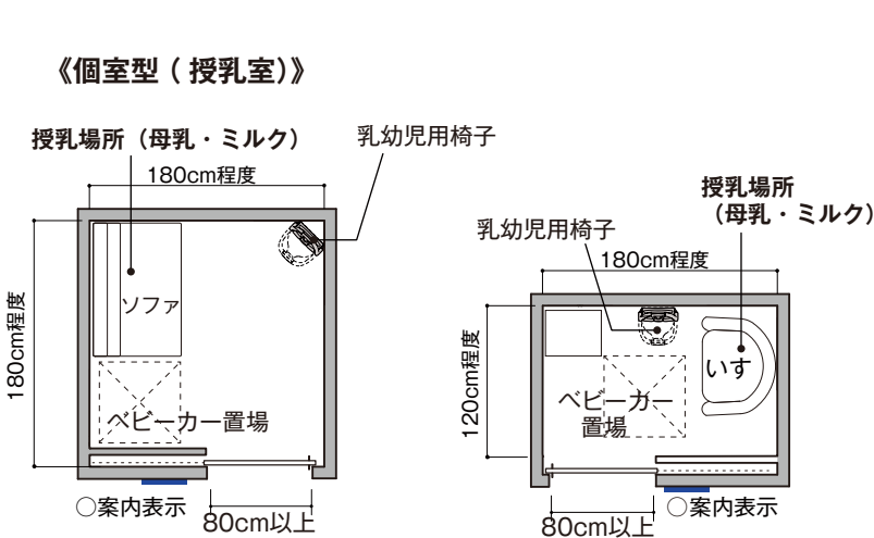
図20-3 授乳室の整備例 (個室型)
