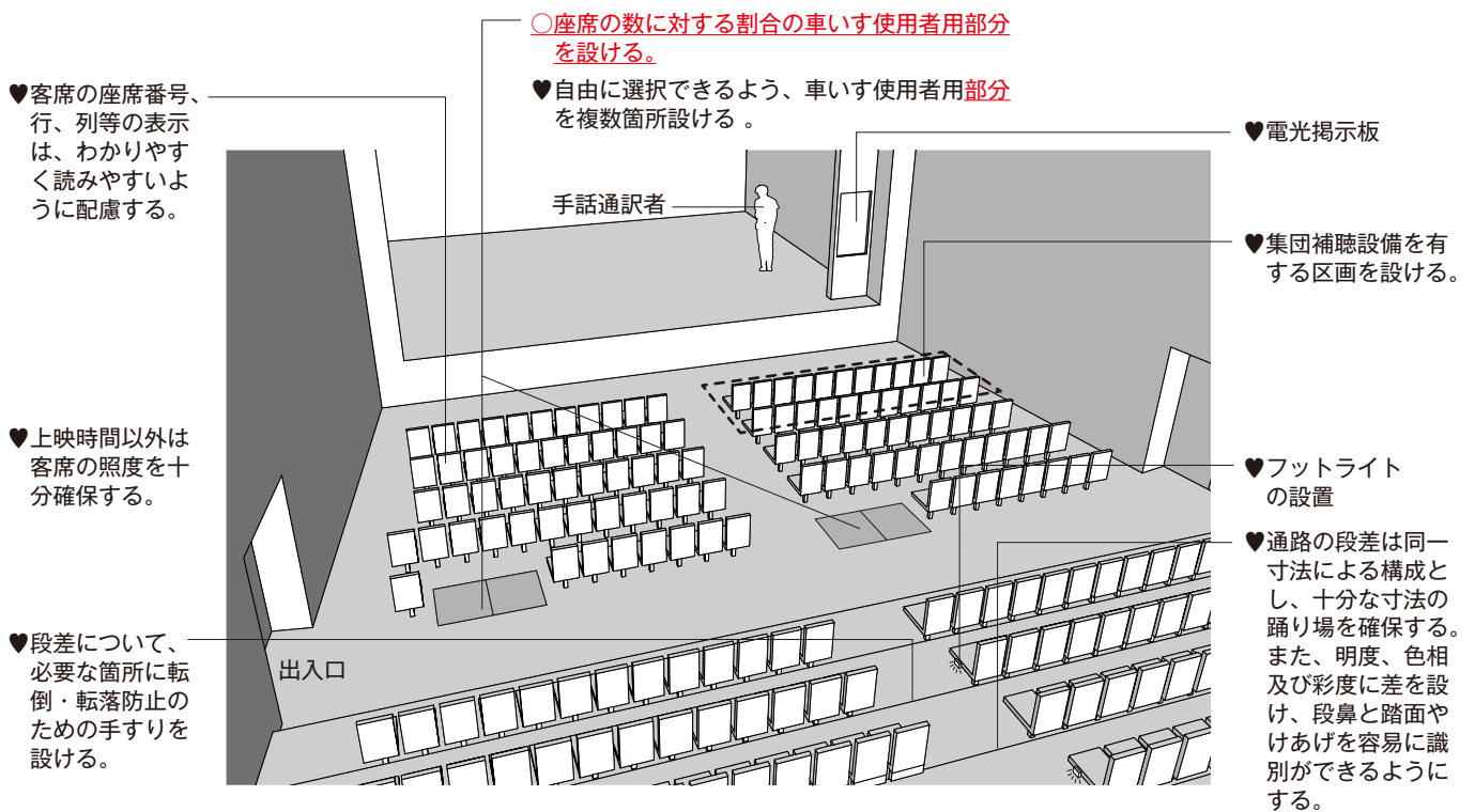
図12-1 客席の整備例
