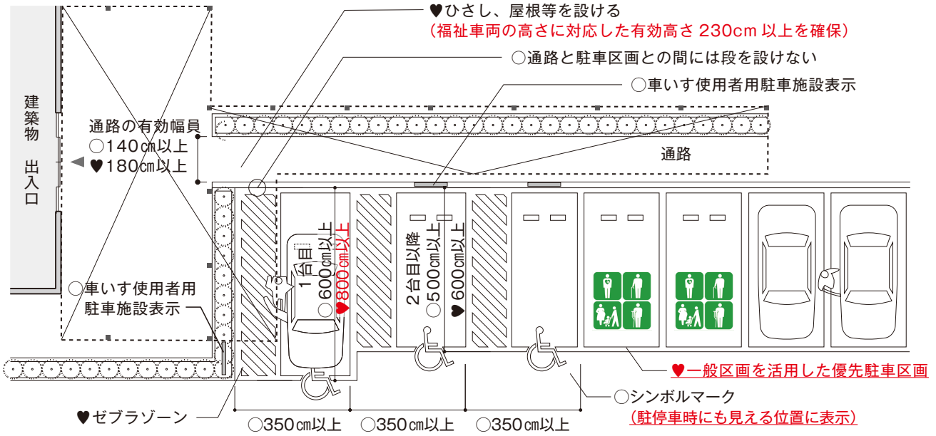
図3-1 自走式駐車場の整備例
