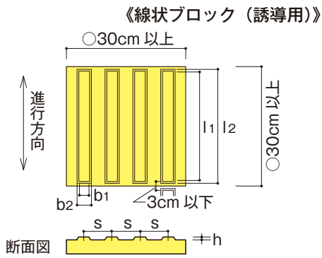
図21-1 線状ブロック等・点状ブロック等の構造
