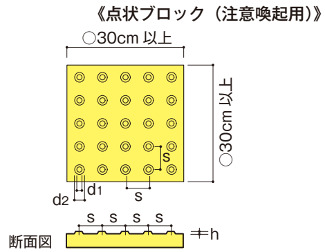
図21-1 線状ブロック等・点状ブロック等の構造
