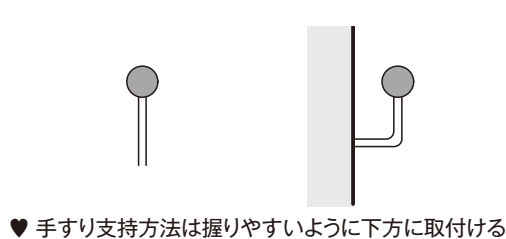
図6-5 手すりの形状、固定方法、端部納まり
