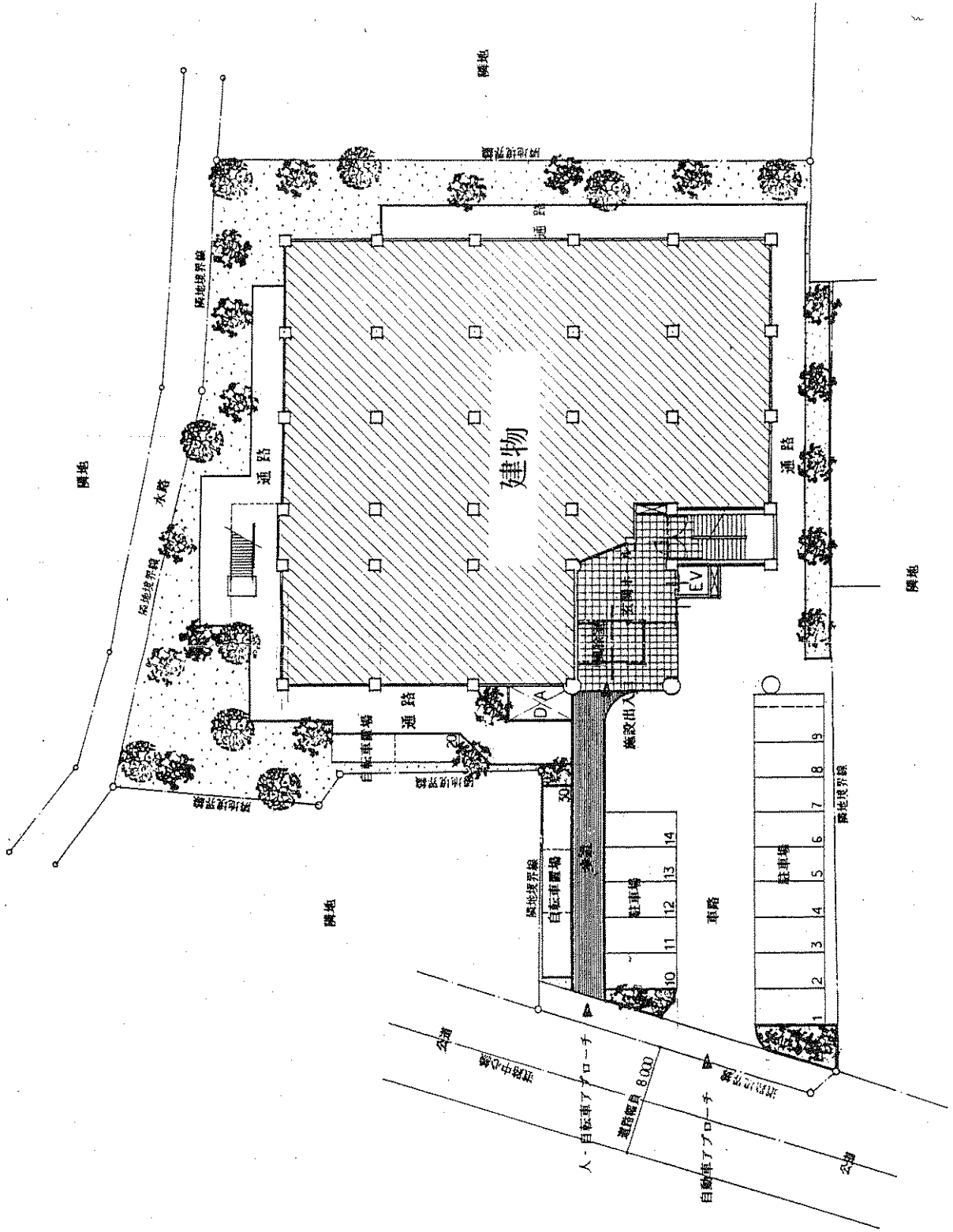
配置図
