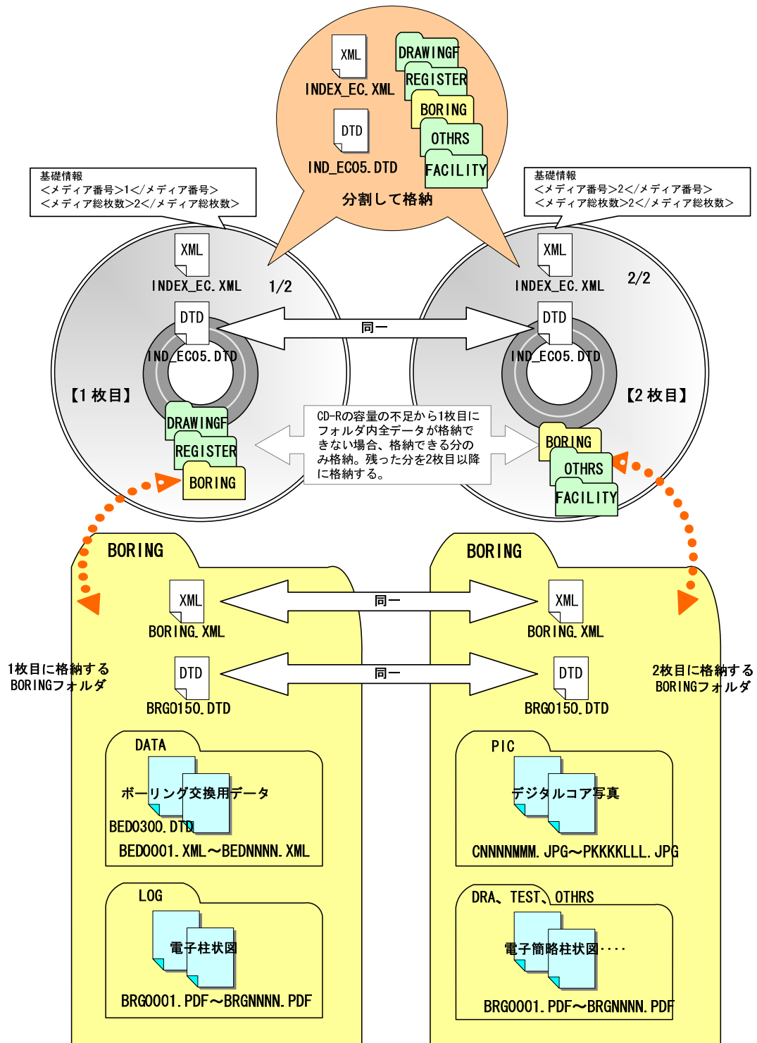
図 5-23 電子媒体が2枚になる場合の作成(例)【フォルダを分割する場合】
