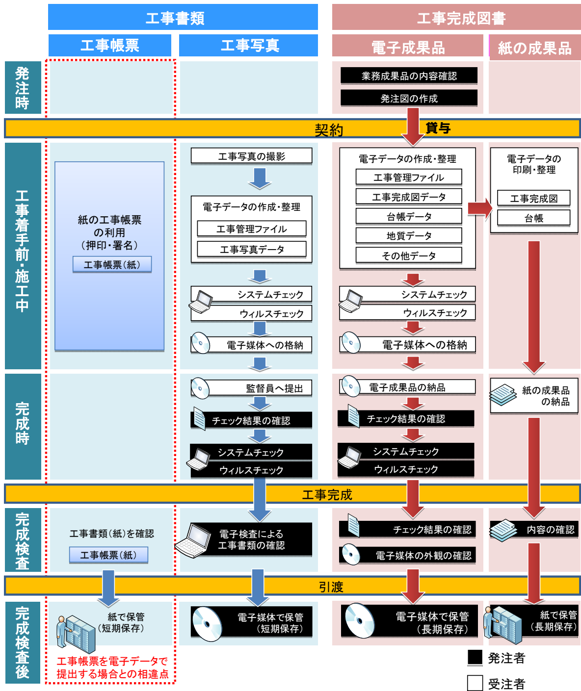
図 2-1 電気通信設備工事における電子納品・電子検査の流れ (紙の工事帳票を利用する場合)
