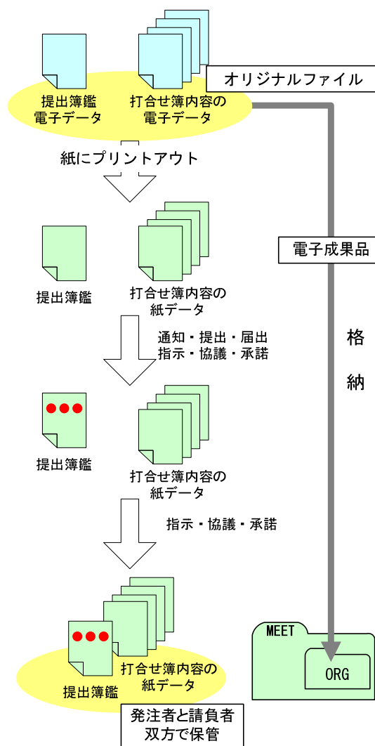
図 7-5 打合せ簿オリジナルファイルの取り扱い（例）
