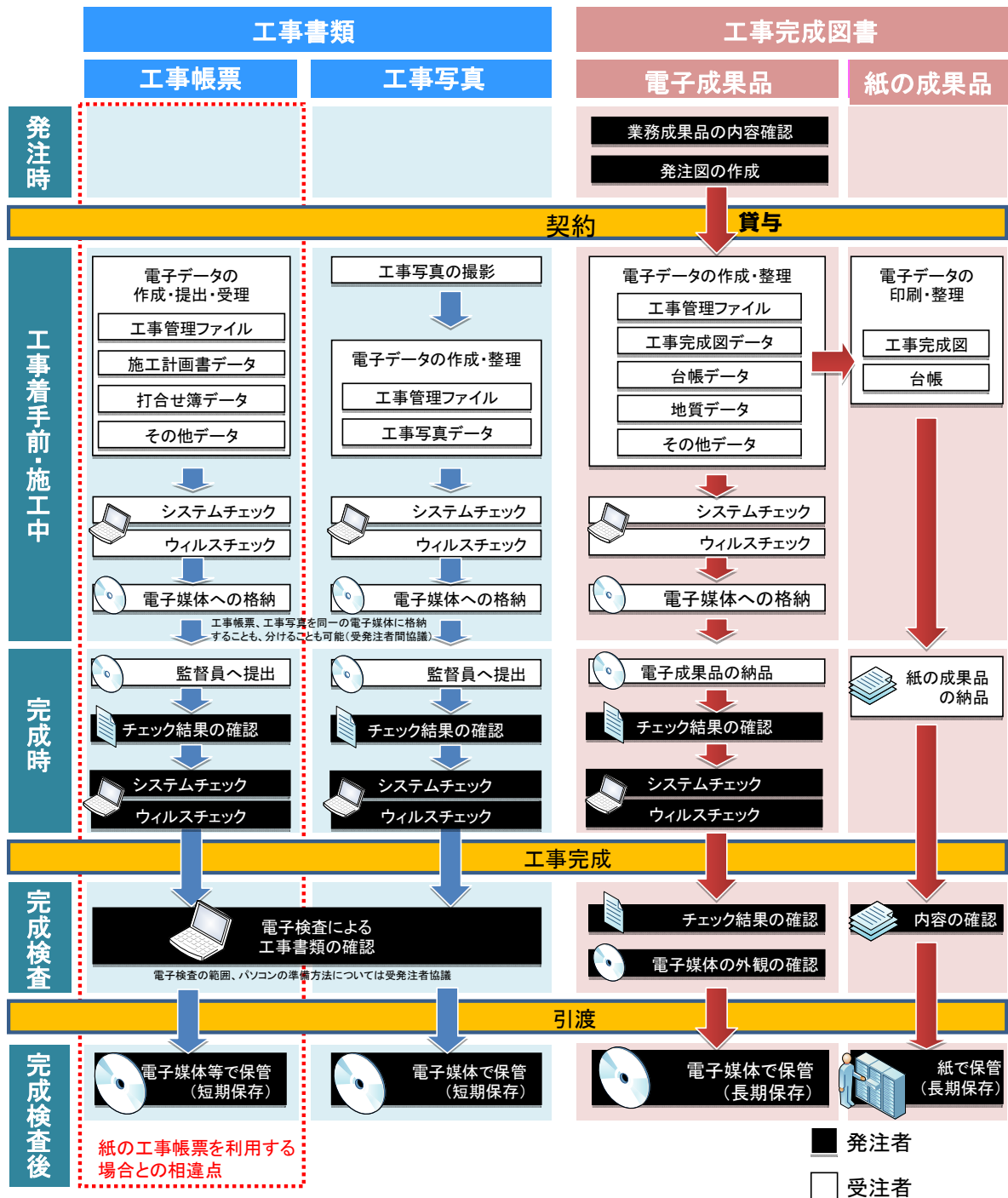
図 2-2 電気通信設備工事における電子納品・電子検査の流れ
