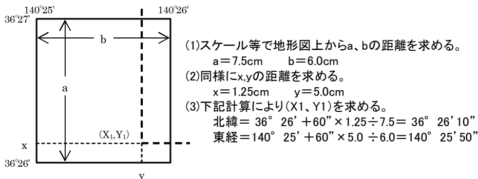
図付 3-4 メッシュ拡大図
