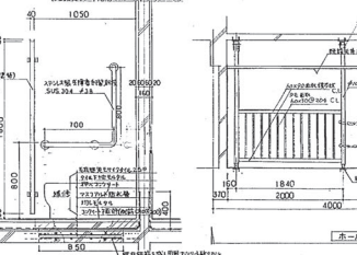
断面図 1/50
