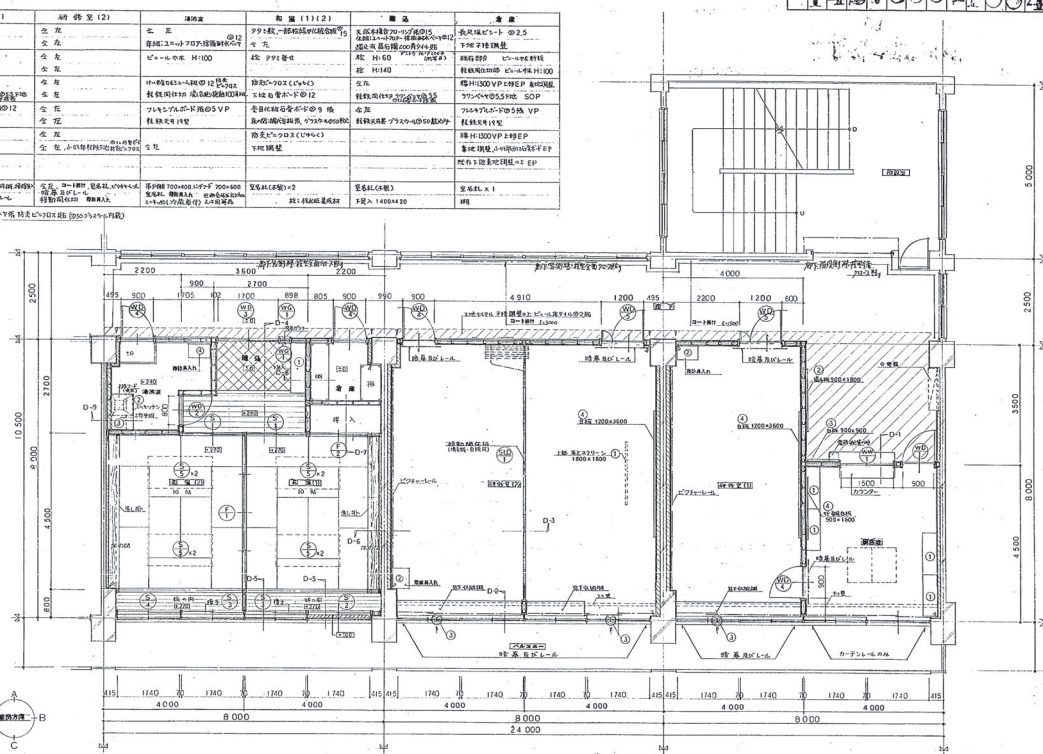
第10図 平面図 (1/50)
