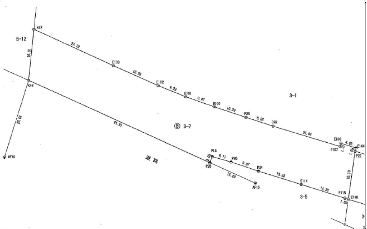
座標求積表
