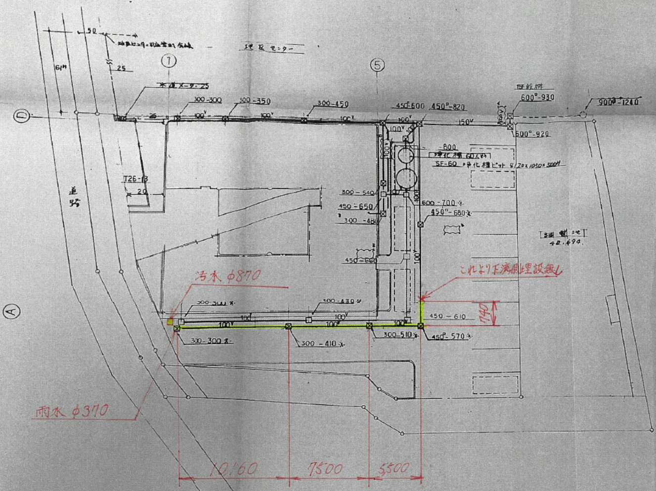
配置図
