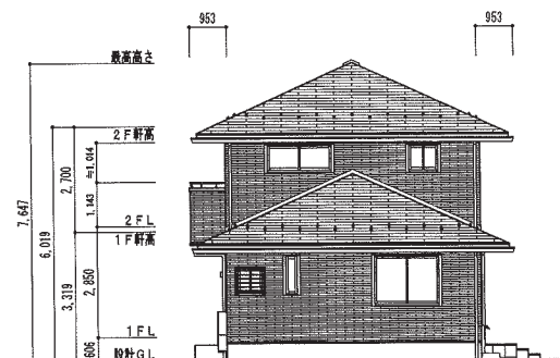
西側立面図
