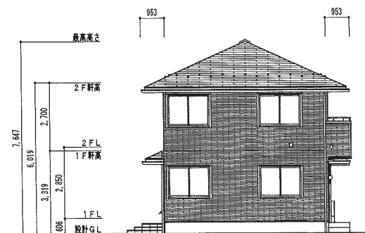
東側立面図
