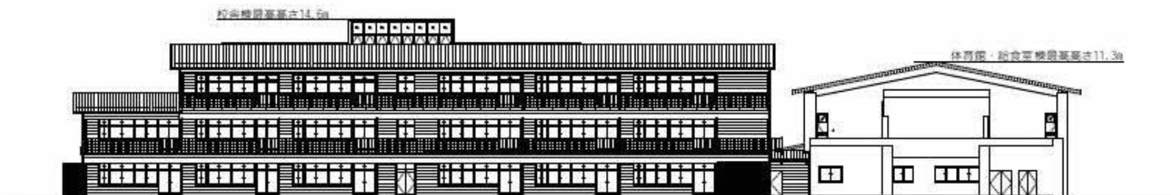
南側立面図
