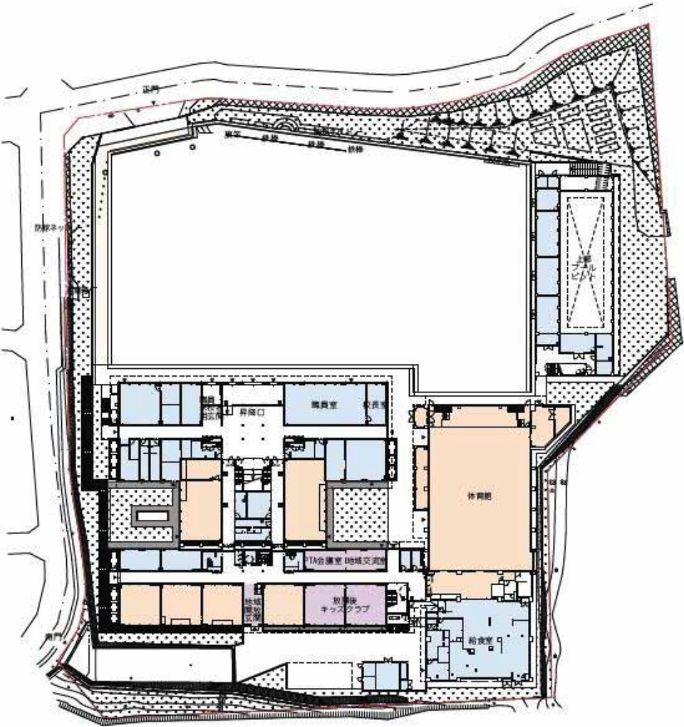
1階平面図
