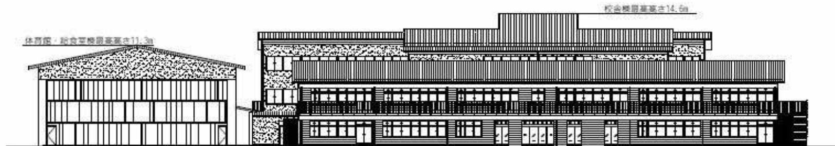
北側立面図
