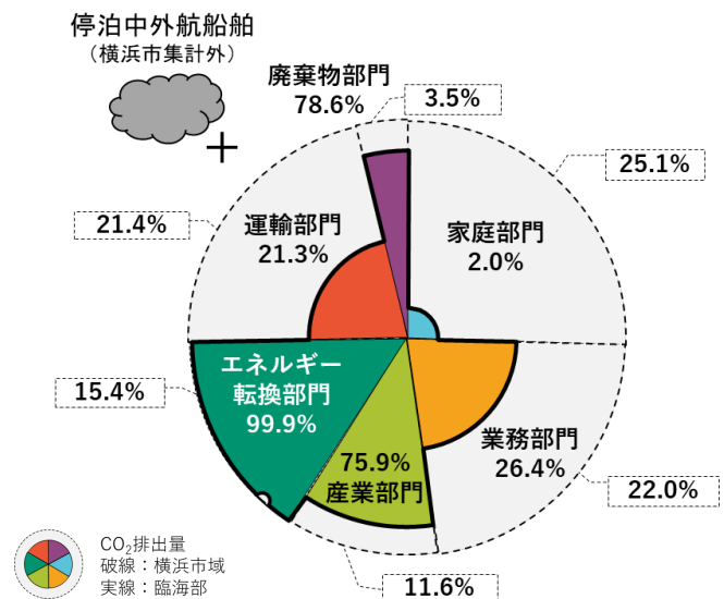
図25 2023年度のCO 2 排出量の推計グラフ
