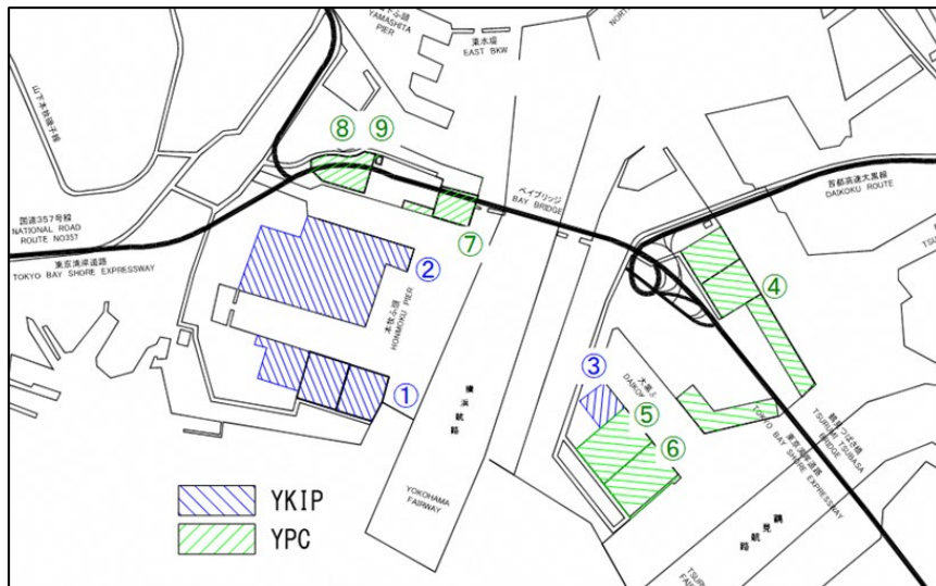
再生エネ由来の電力を供給する施設
