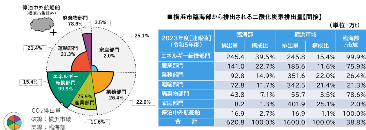
図44 横浜市臨海部から排出される二酸化炭素排出量（間接排出量）
