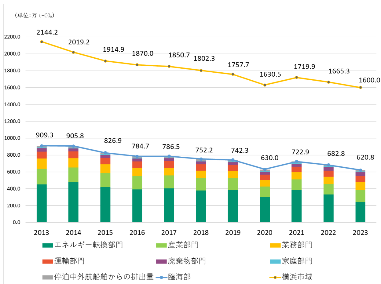
図26 横浜地域と横浜市臨海部のCO 2 排出量の推移（停泊中外航船舶からの排出量含む）
