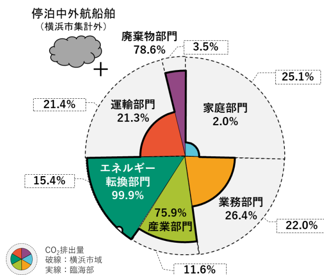
図25 2023年度のCO 2 排出量の推計グラフ
