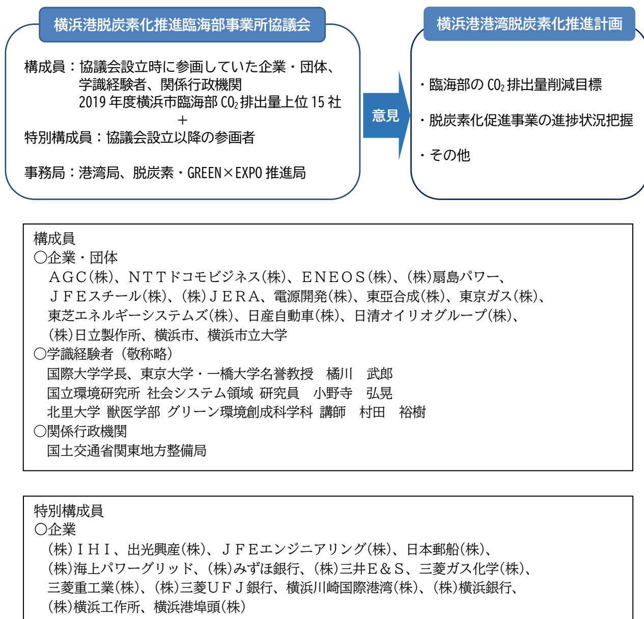
図35 横浜港脱炭素化推進臨海部事業所協議会の実施体制
