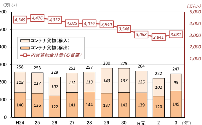
図13 内貨コンテナ貨物量の推移
