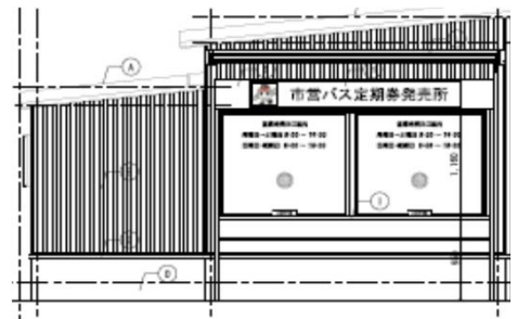
新設建物計画図
