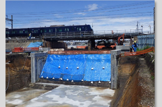
工事状況 (擁壁築造)
