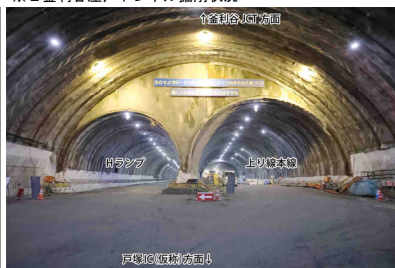
※2 金沢谷庄戸トンネル掘削状況
