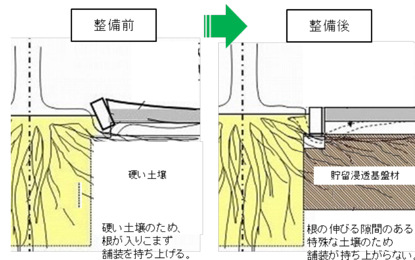
グリーンインフラ整備（根上り対策工）概念図
