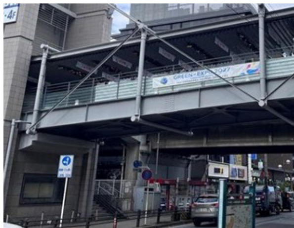
青葉台駅前第一歩道橋（青葉区）： 桁を支える下部工の台座部を拡幅
