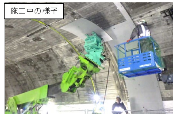
相武隧道(金沢区)：鋼板内巻工法による補強を実施
