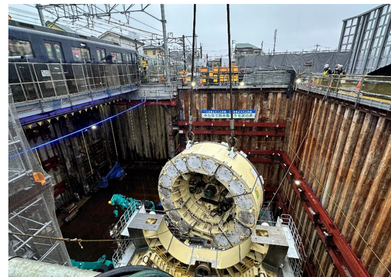
シールドマシンの組立状況
