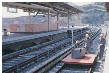
地下鉄上永谷駅工事(港南区) 1976年04月 7347
