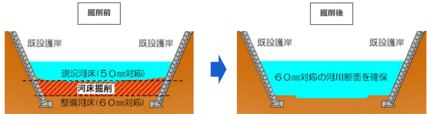
<時間降雨量60mm対応の河川整備のイメージ>
