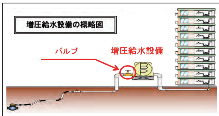
増圧給水設備の概略図
