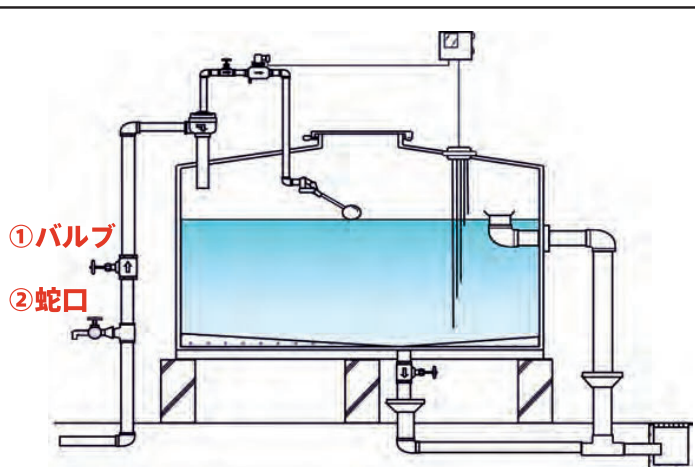
標準的な受水槽の断面と受水槽廻りの配管
