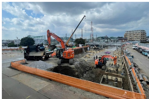
▲新築工事（土工事）
