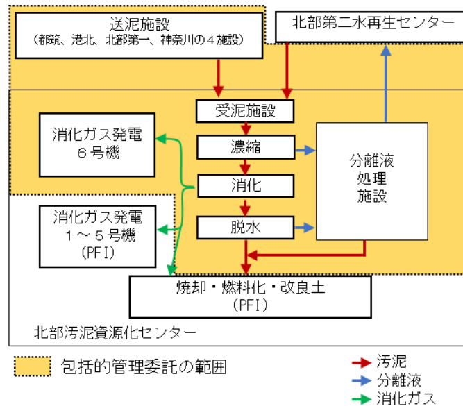
図1 北部汚泥資源化センター包括的管理委託範囲の概要図
