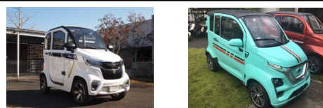
図 出展車両（e-moシリーズ）
