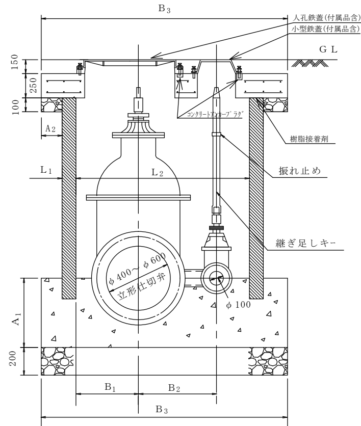
断面図
