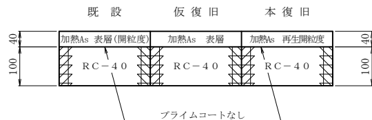
P a タイプ 歩道舗装（自動車乗入れ部） 個人住宅用 2 t 未満
