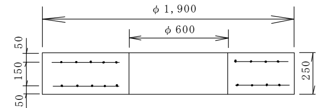
配筋図 (床版断面図)
