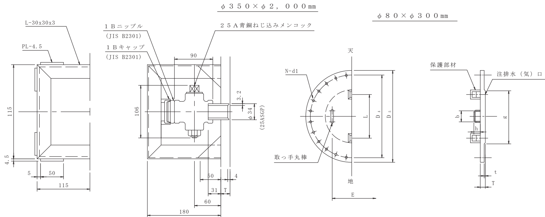
F 1 2 (最高許容圧力1.2MPa, 使用圧力0.74MPa (=7.5kgf/cm 2 ) 単位: mm
