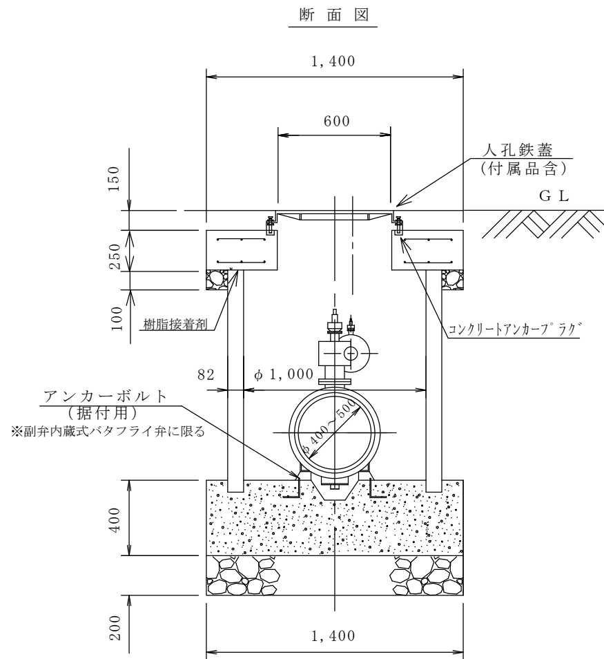
材 料 表
