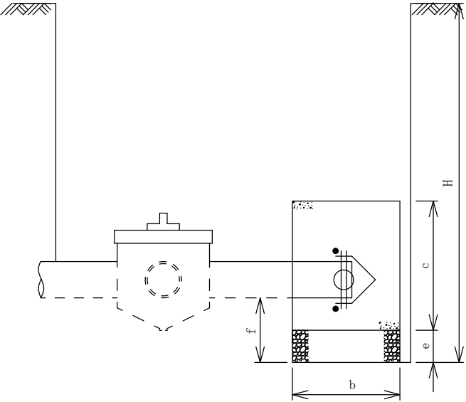
断 面 図
