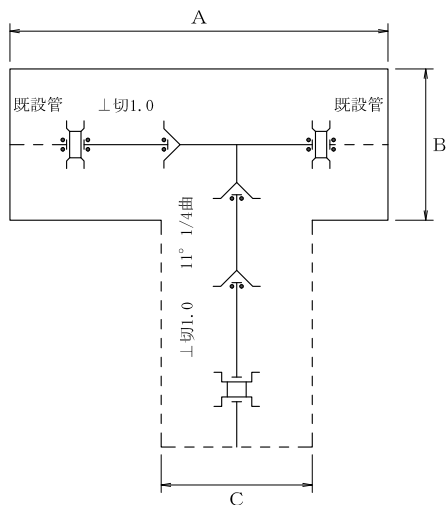
平面図 ( 2 )
