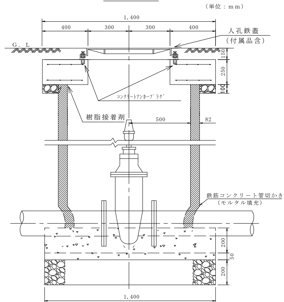
断 面 図
