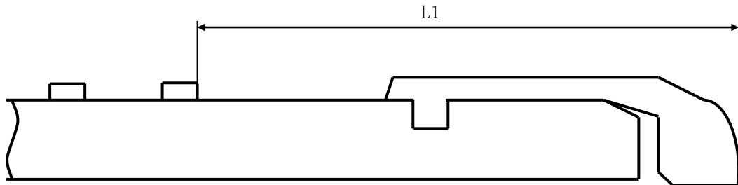
図 2-5 GX形ダクタイル鋳鉄管の白線表示位置
