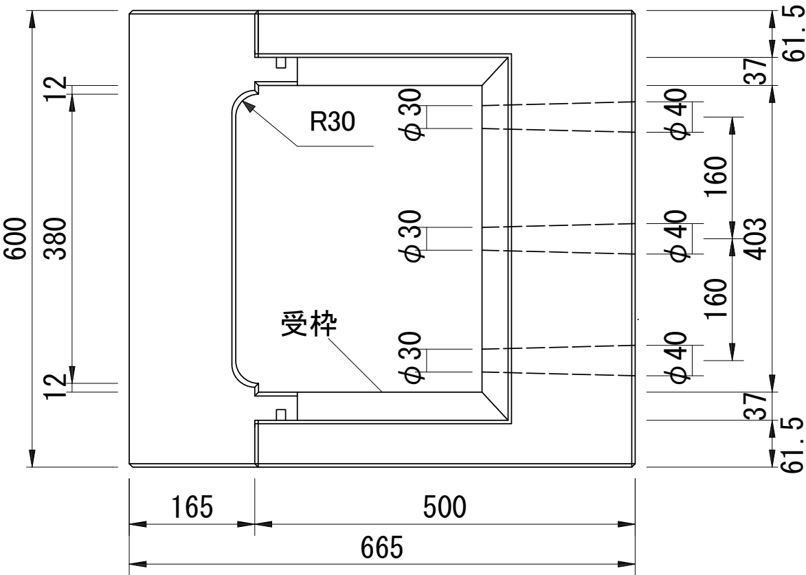
側面図
