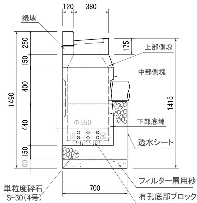
B-B 断面図
