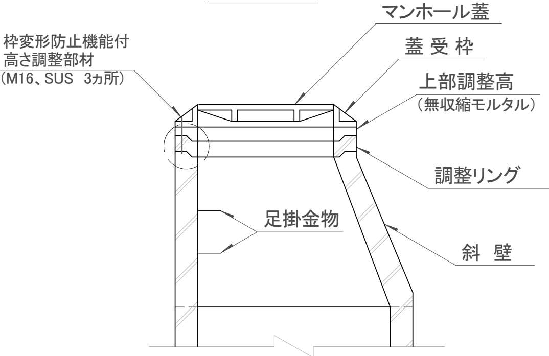
断面図
