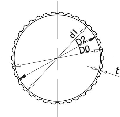
カラー部詳細図
