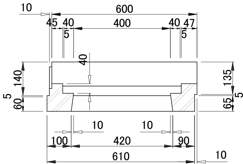
A-A 断面図
