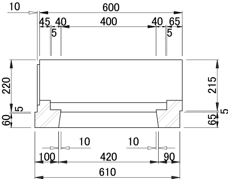
B-B 断面図
