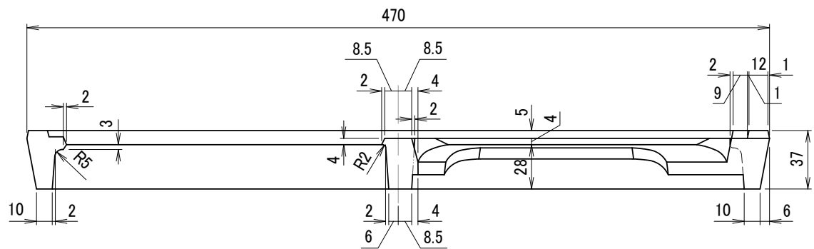
A-A断面図
