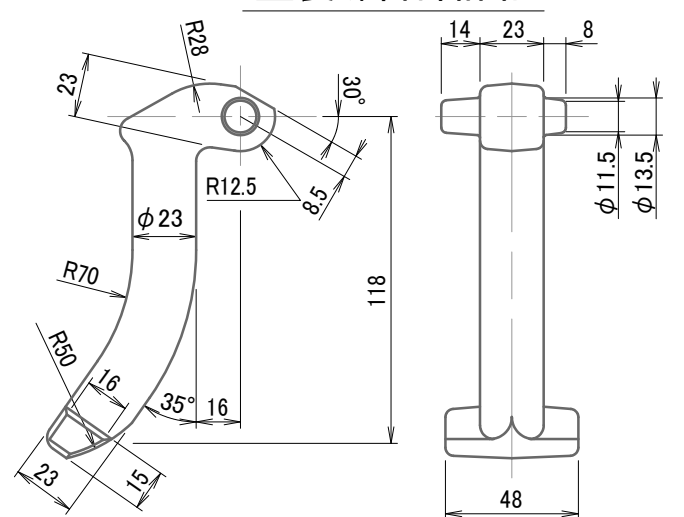
蝶番金物詳細
