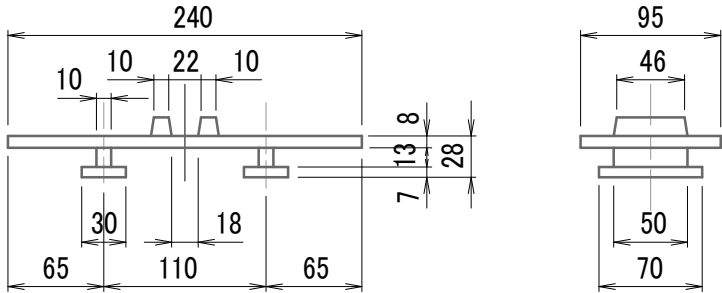
ずれ止め詳細
