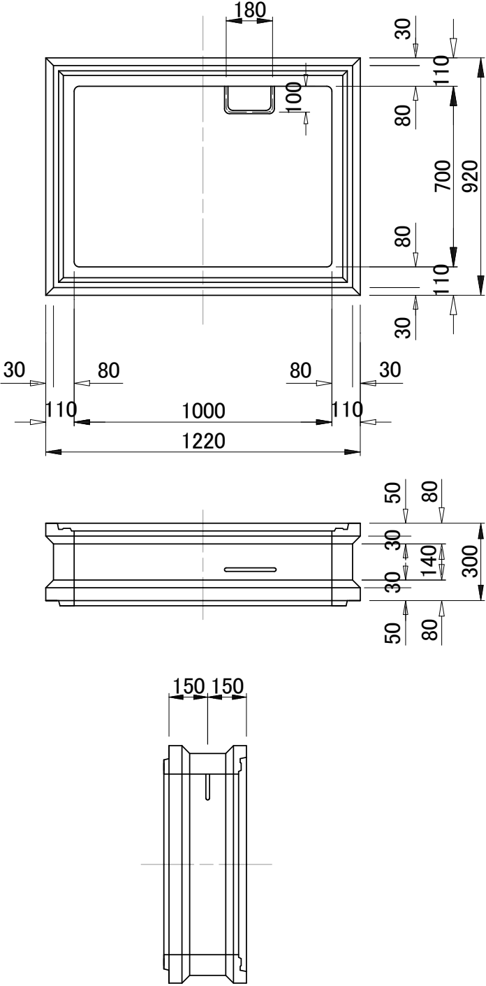
Dブロック構造図
