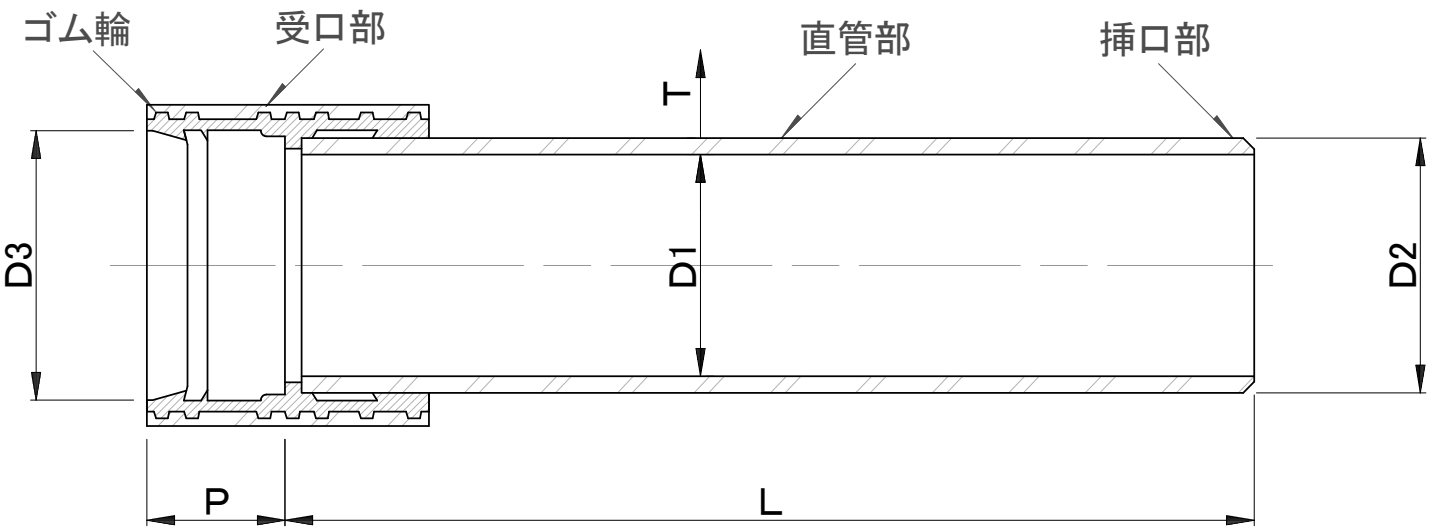
直 管(D形)
