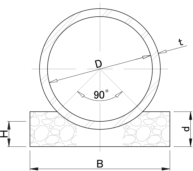
砕石 90° 基礎
