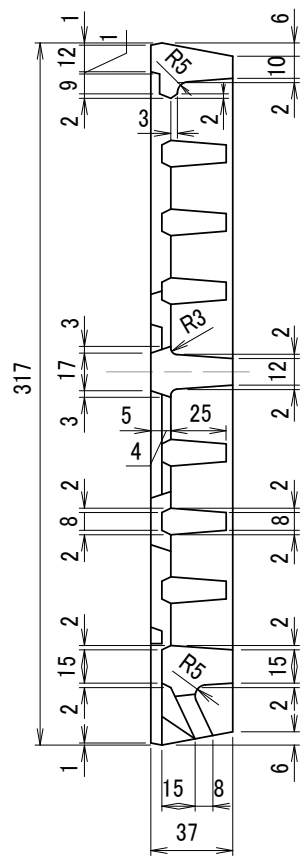
B-B断面図
