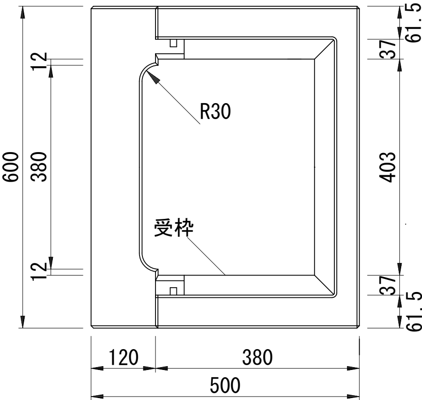
側面図
