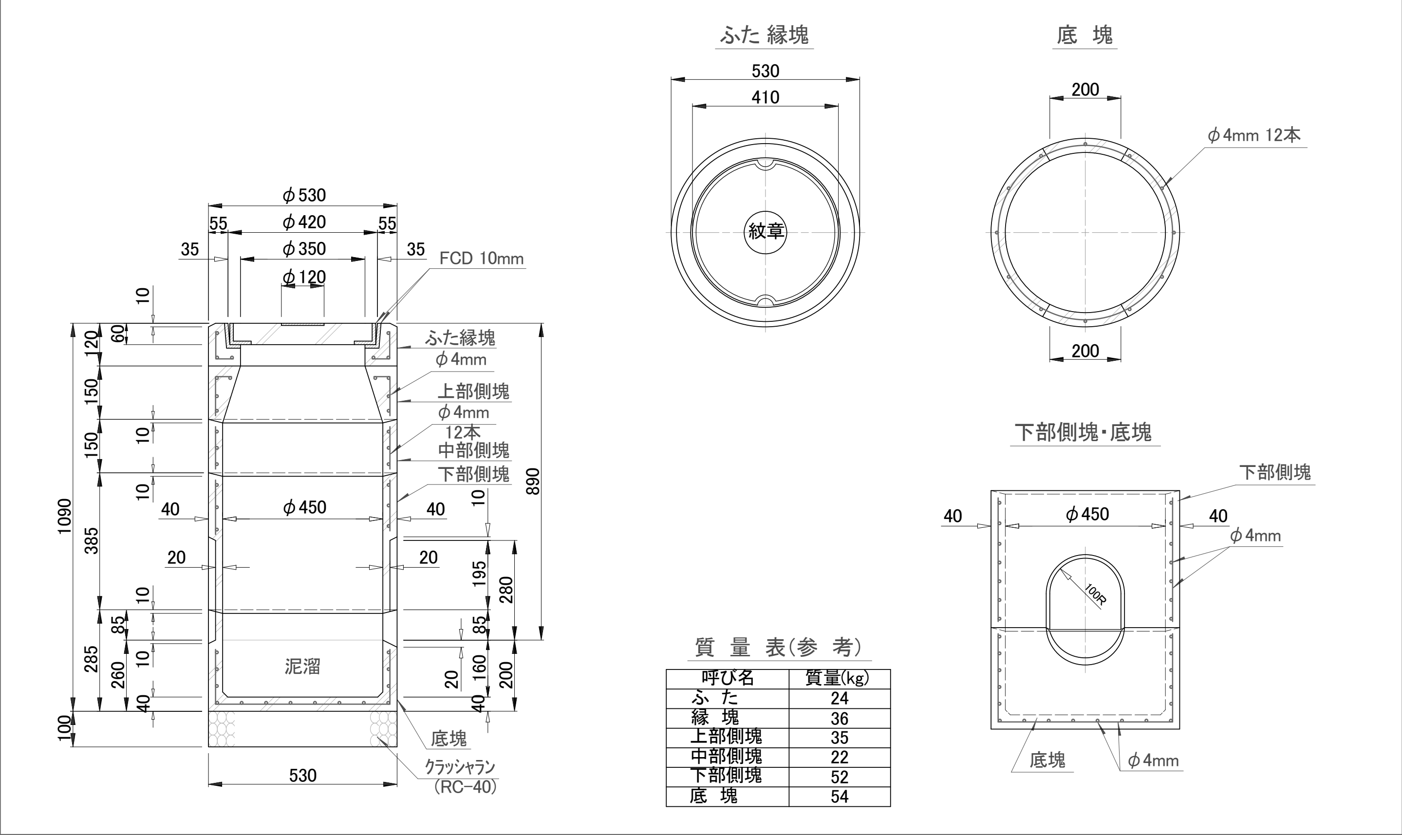
タイプ7接続雨水枡構造図 (φ450)(宅地外)
