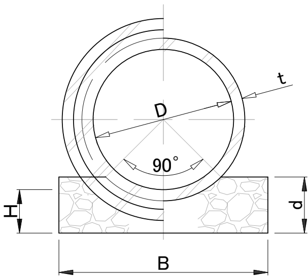
砕石 90° 基礎
