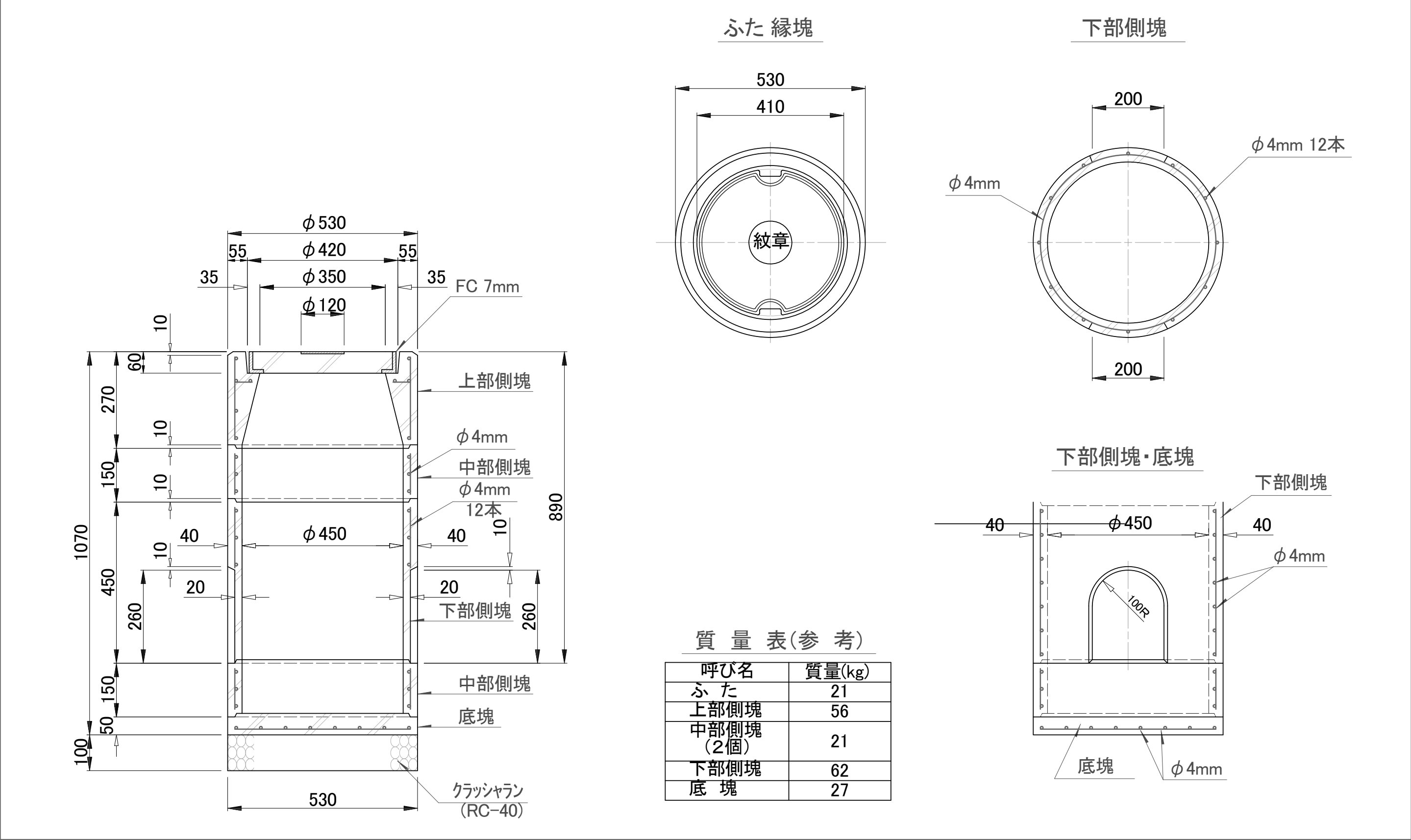
特記事項 タイプ10接続雨水柵構造図 (φ450)
