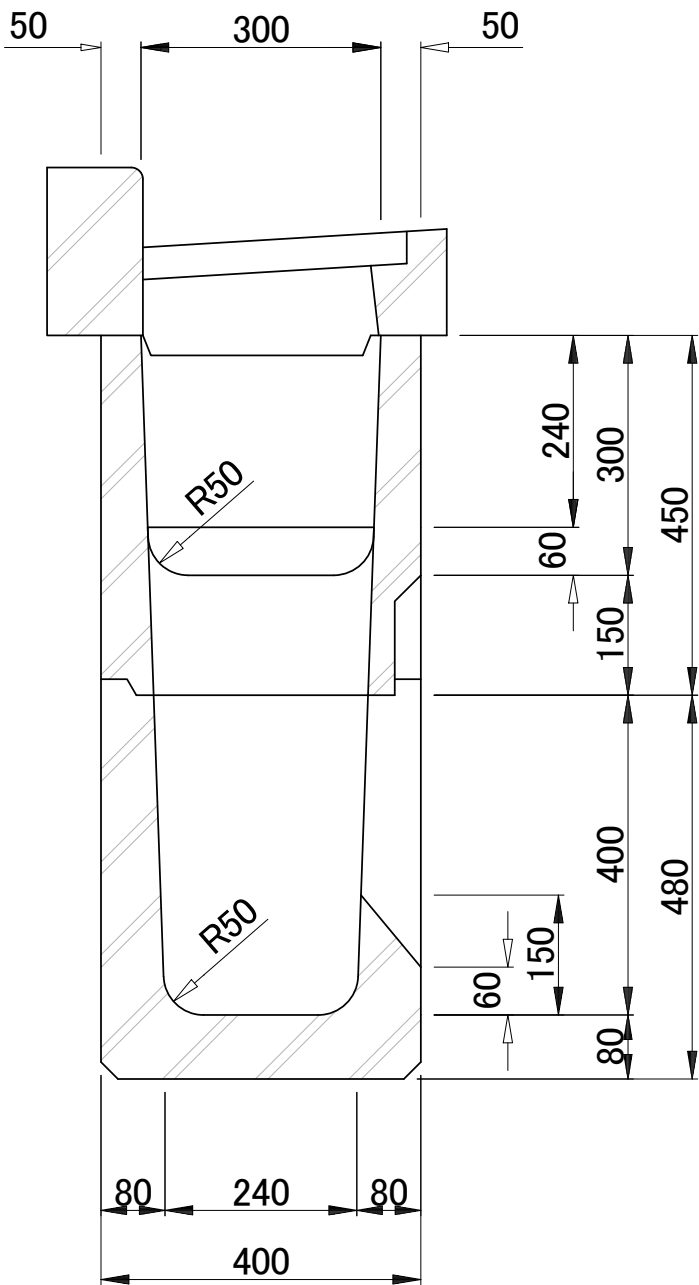
A-A 断面図
