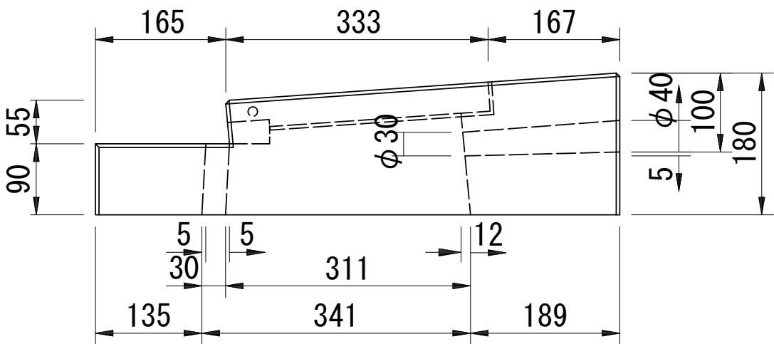
側面図
