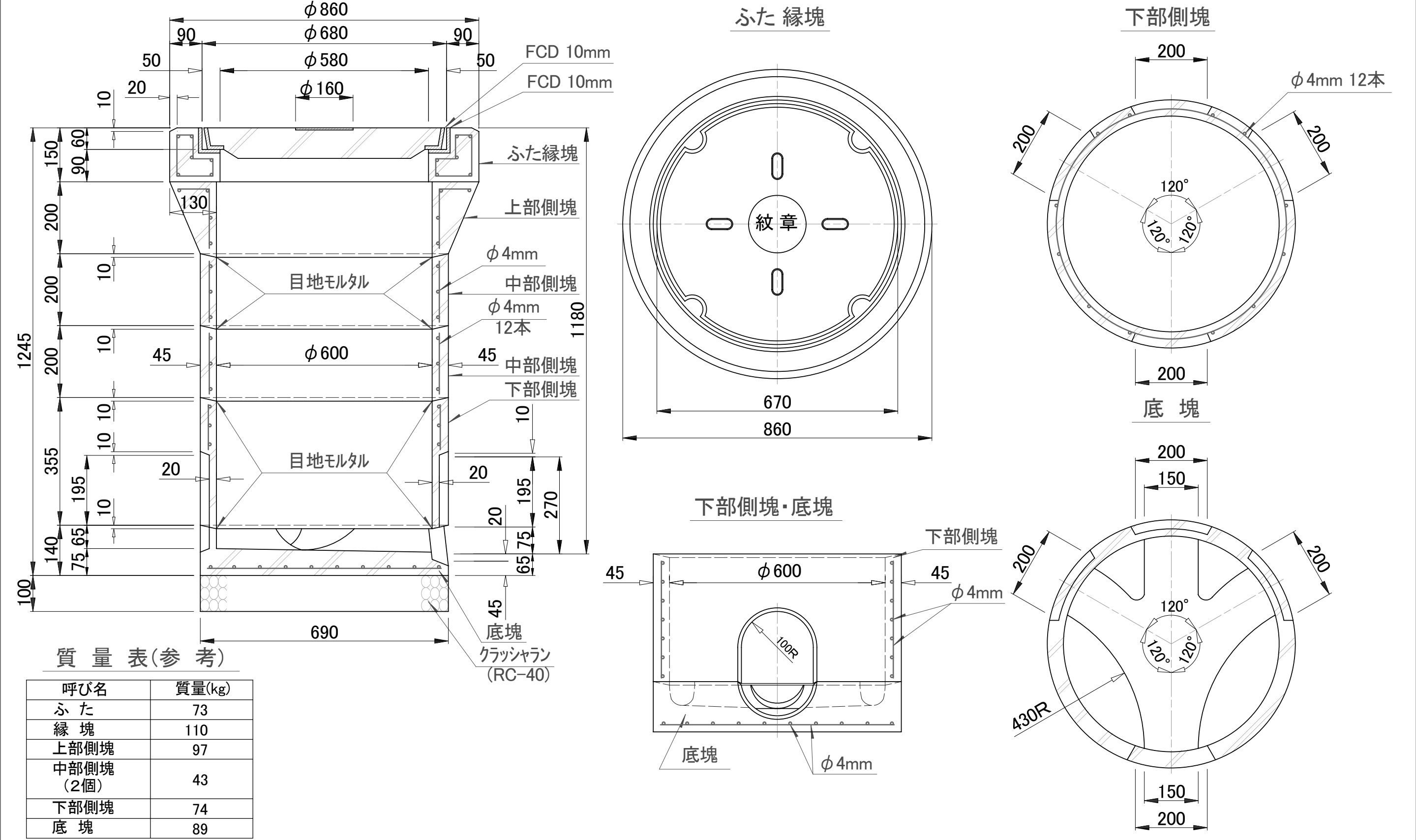
特記事項 タイプ2接続汚水枡構造図 ( \phi 600 )
