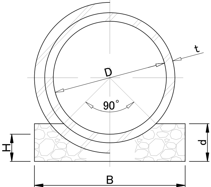
砕石 90° 基礎
