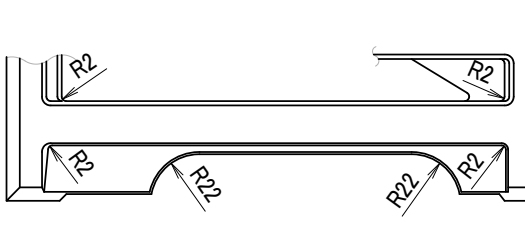
裏面図
