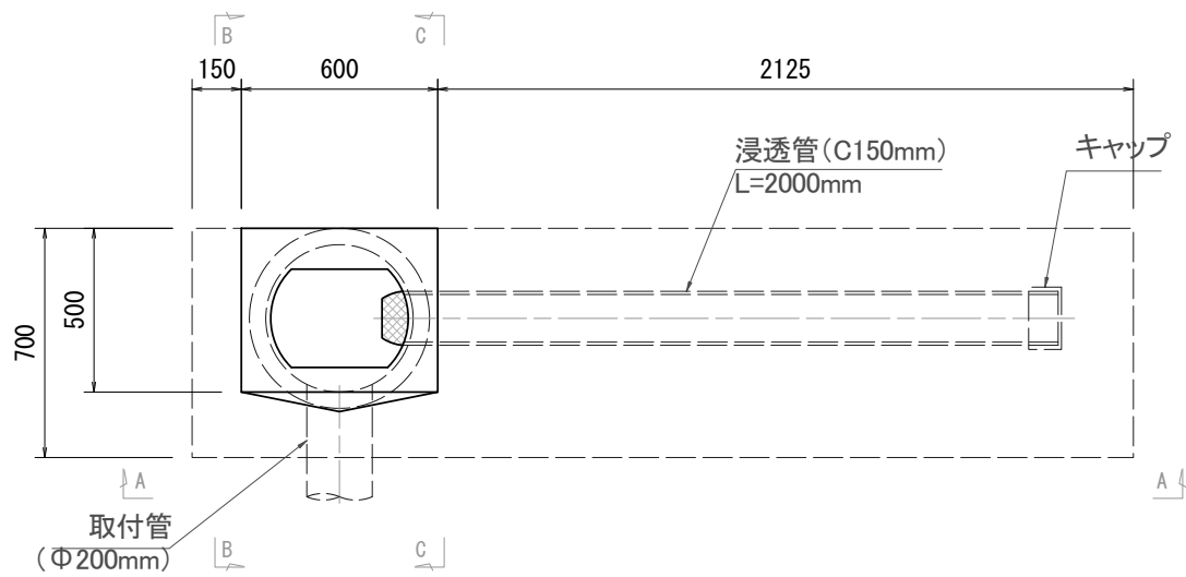
平面図
