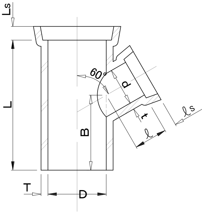
寸 法 表
