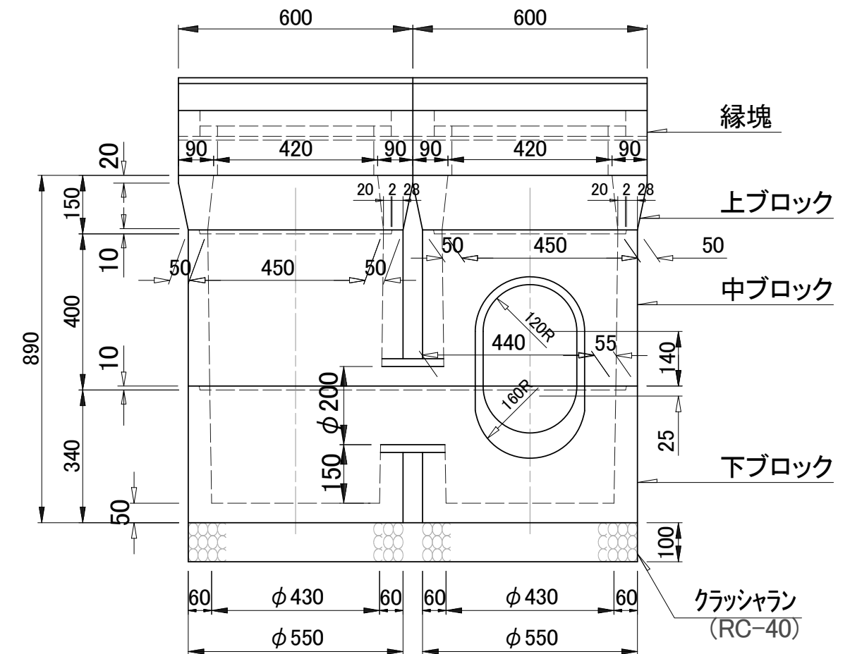
側 面 図
