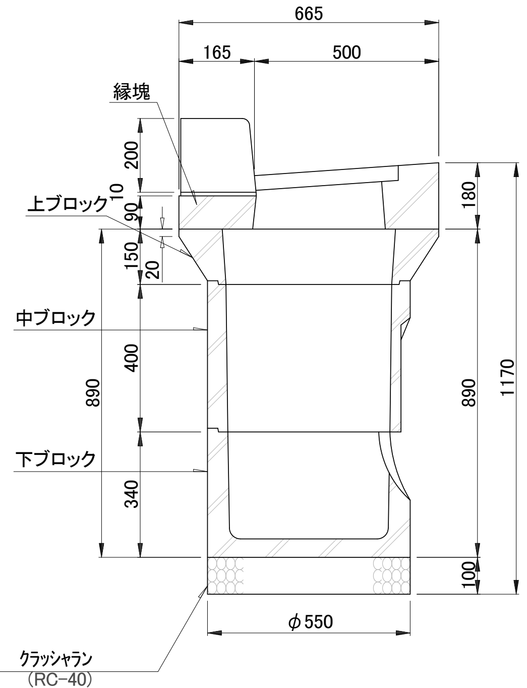
A-A断面図
