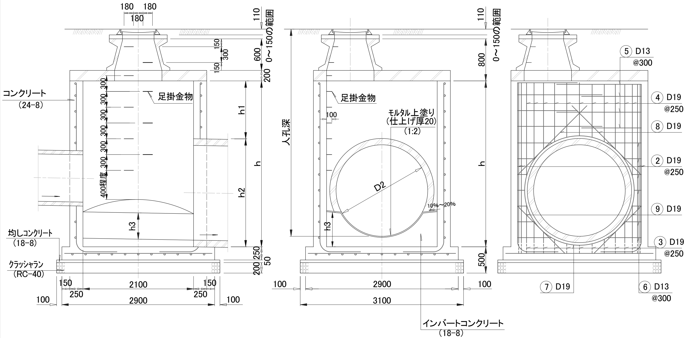
縦断面図
