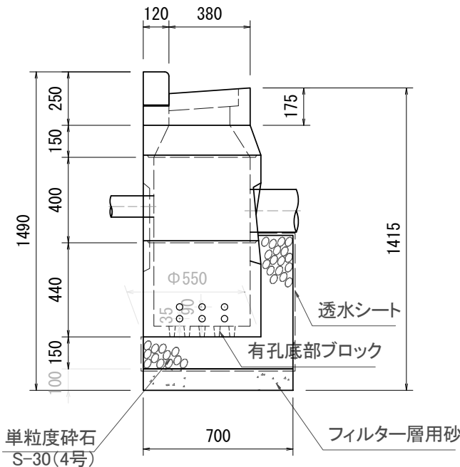
B-B 断面図
