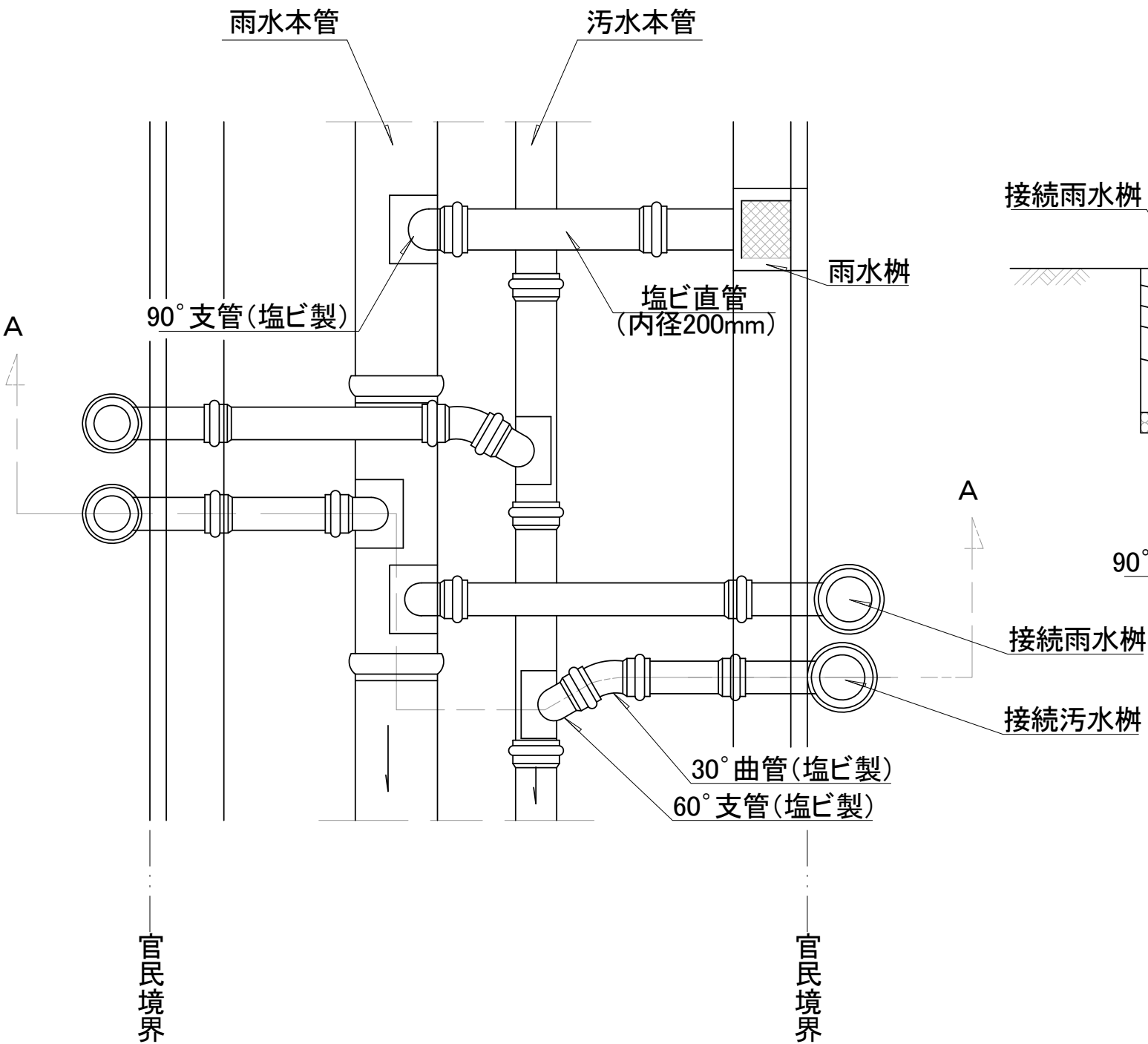
平面図
