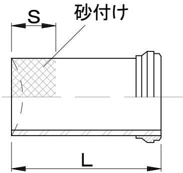
挿口短管
