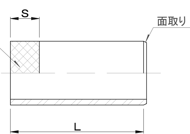
ます取付け継手 (略号 MSB)
