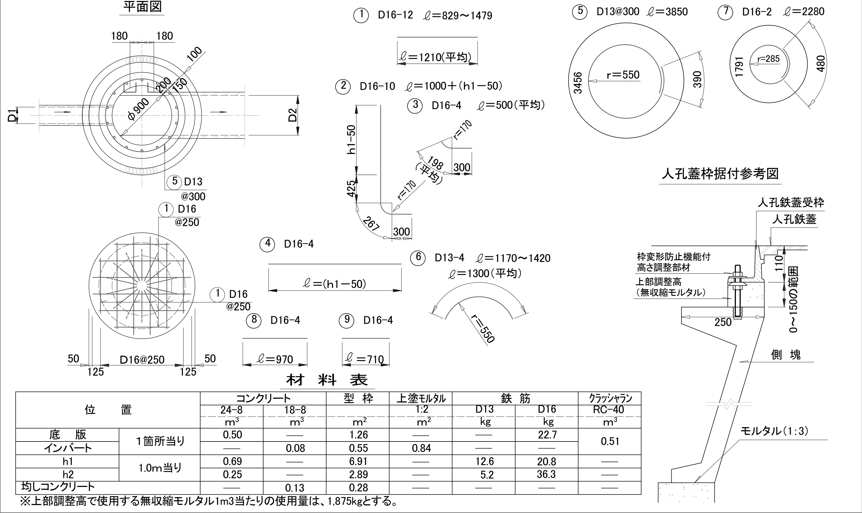
第1種人孔構造図(2)
