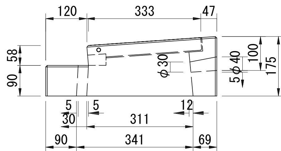
側面図
