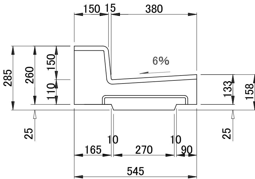
正面図
