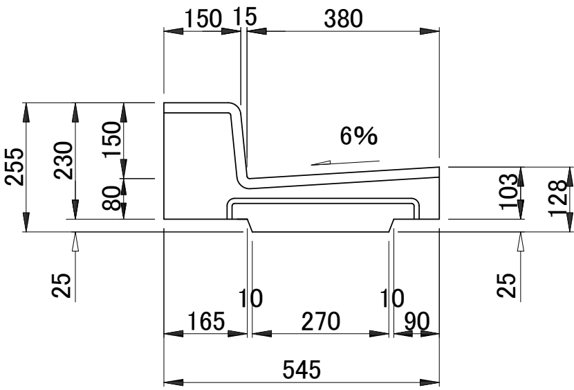
正 面 図
