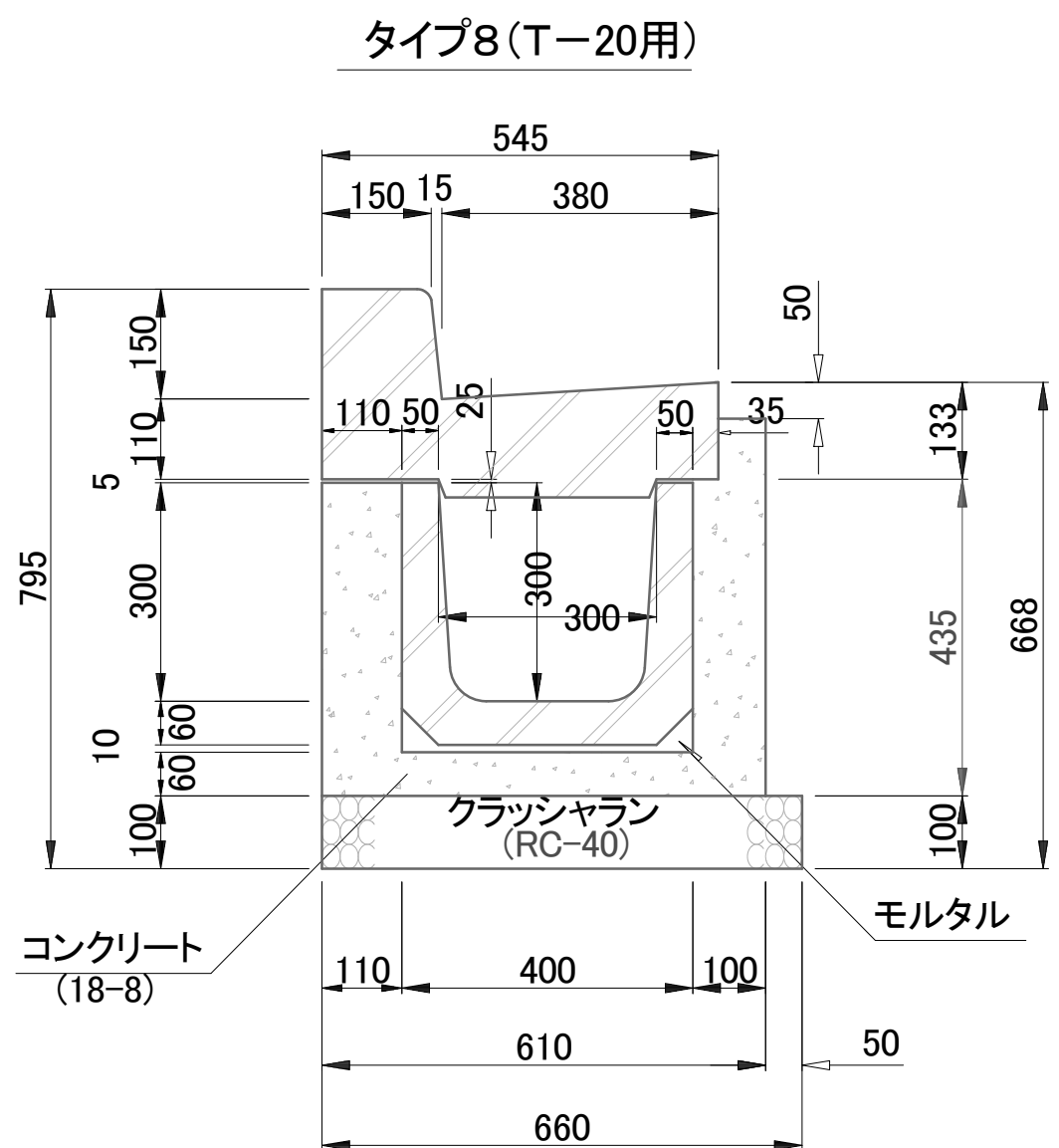
材 料 表
