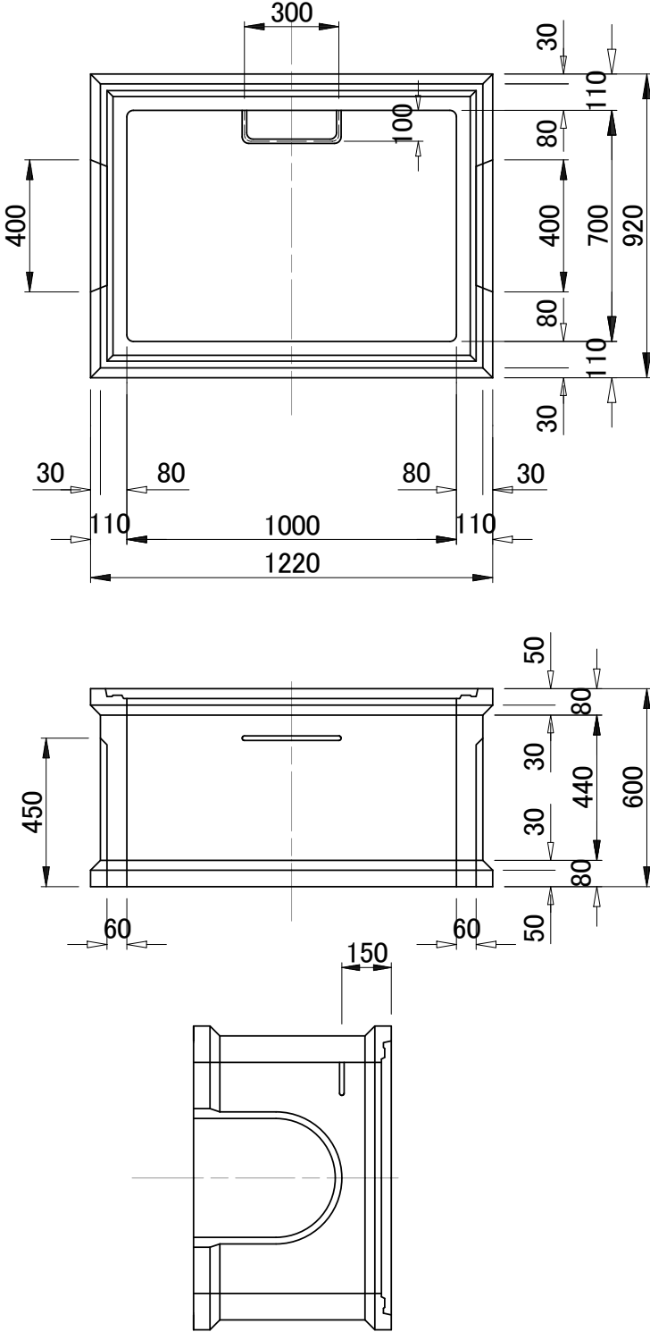
Eブロック構造図
