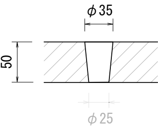
有孔底部ブロック孔詳細図
