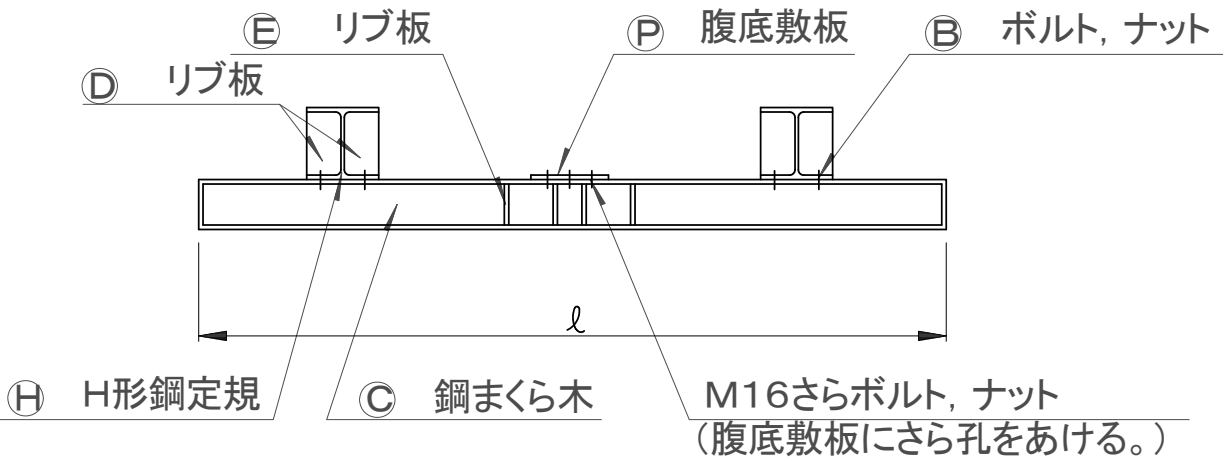
正 面 図
