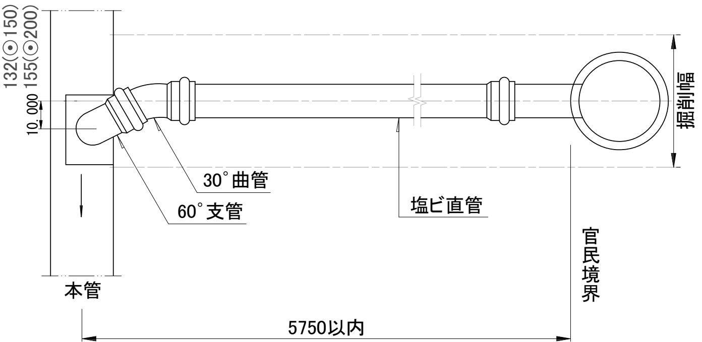
本管(硬質塩化ビニル管)－ 取付管(硬質塩化ビニル管)
