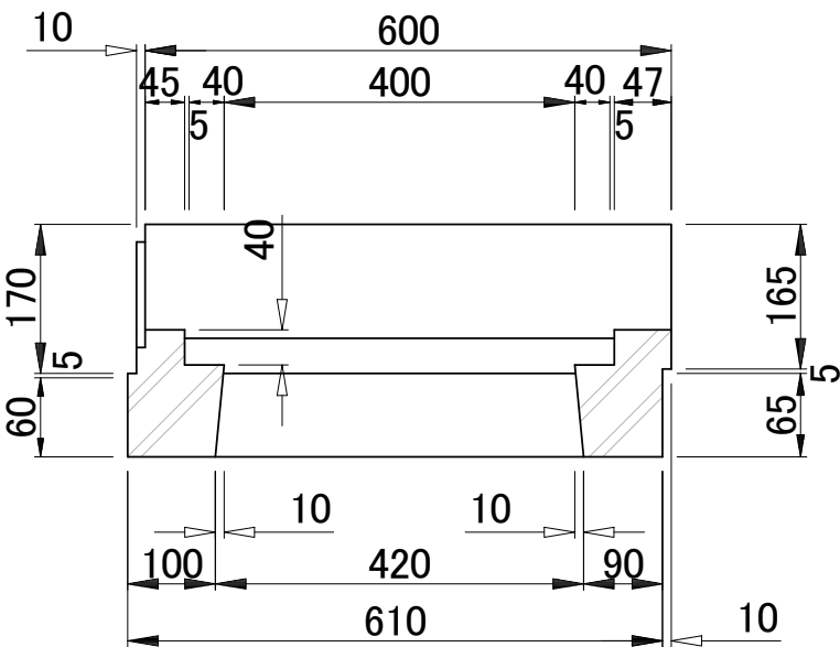
A-A 断面図
