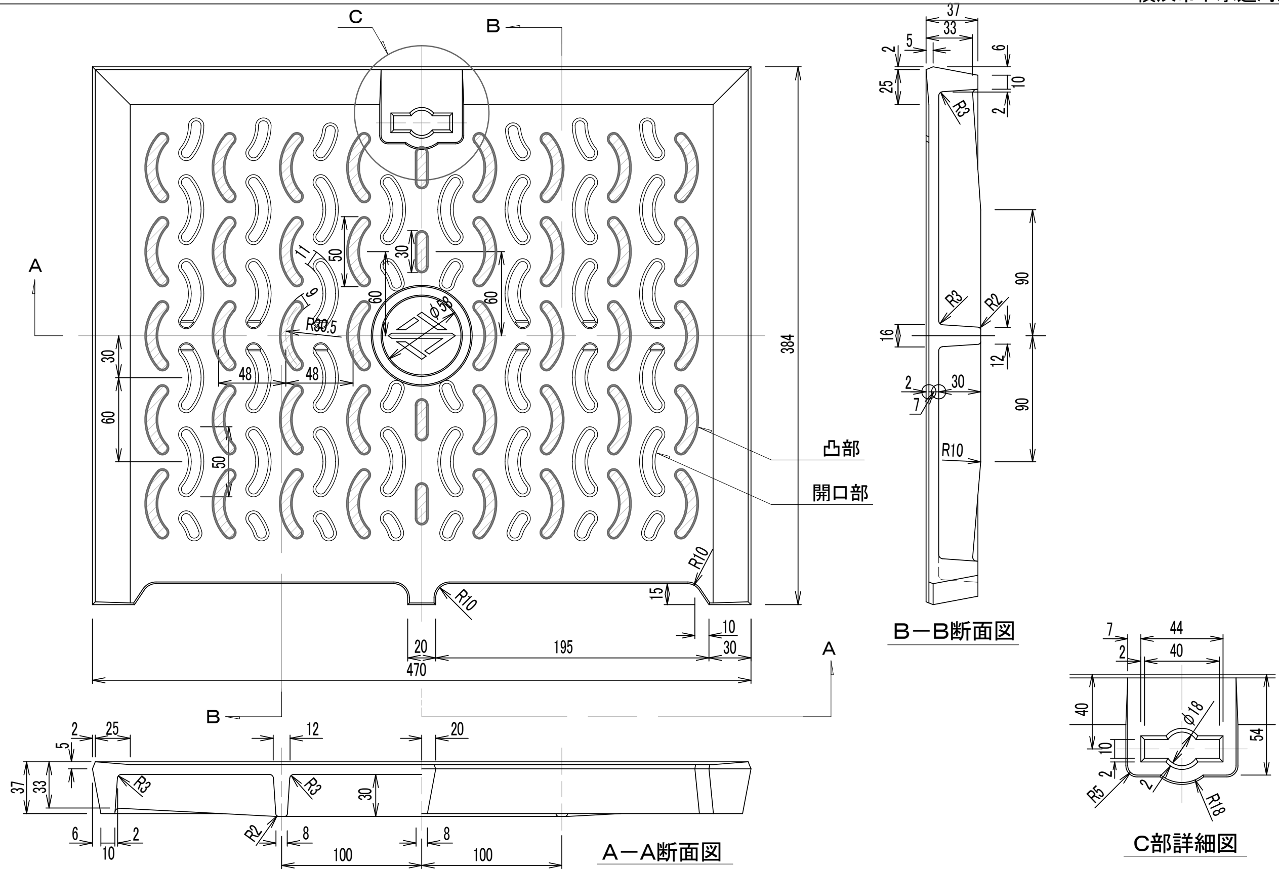
雨水枳蓋(タイプ1用)構造図
