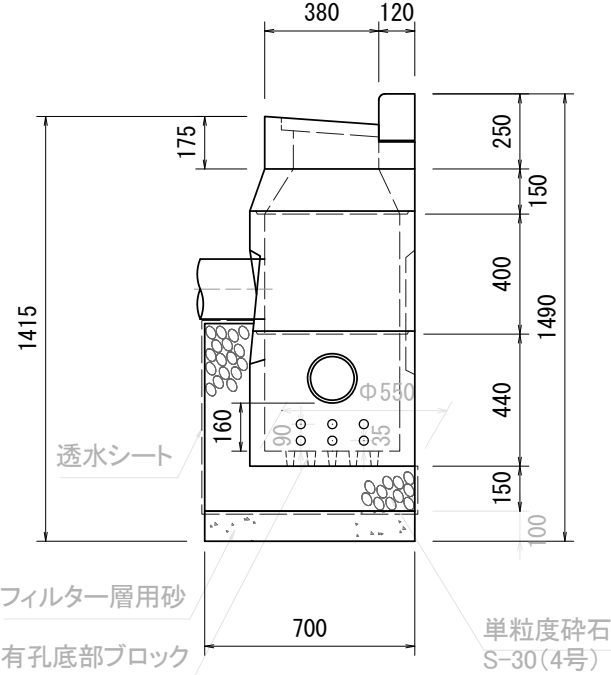
C-C 断面図
