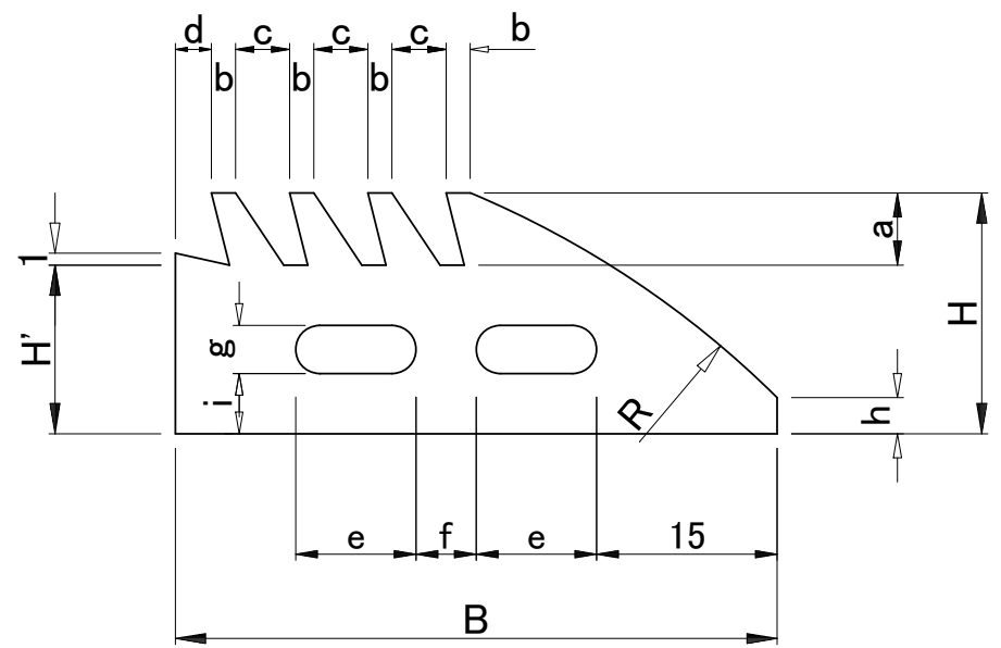
寸法表
