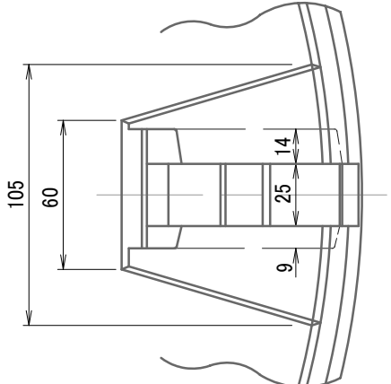
蓋裏蝶番部詳細
