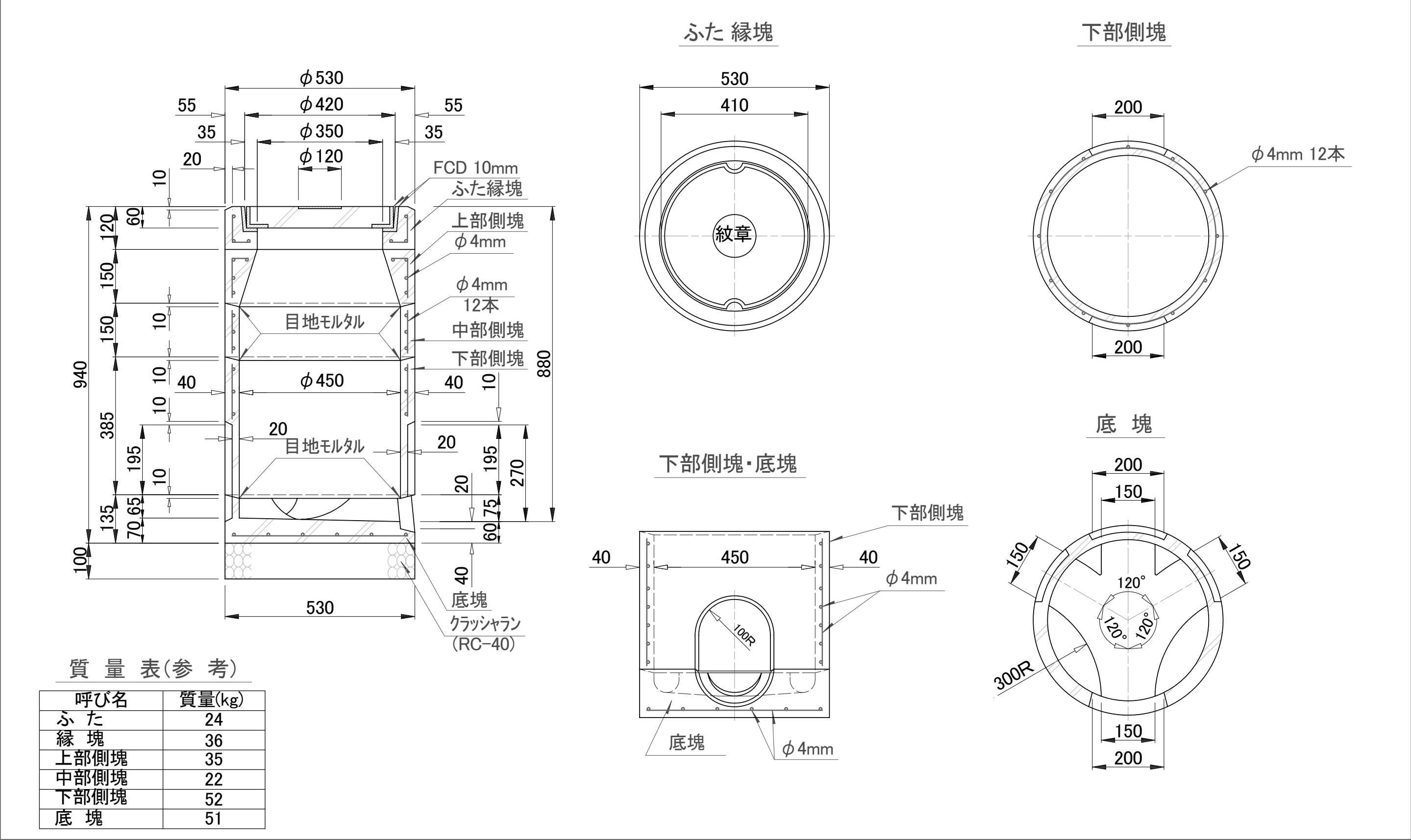
タイプ1 接続汚水枡構造図 (φ450)(宅地外)
