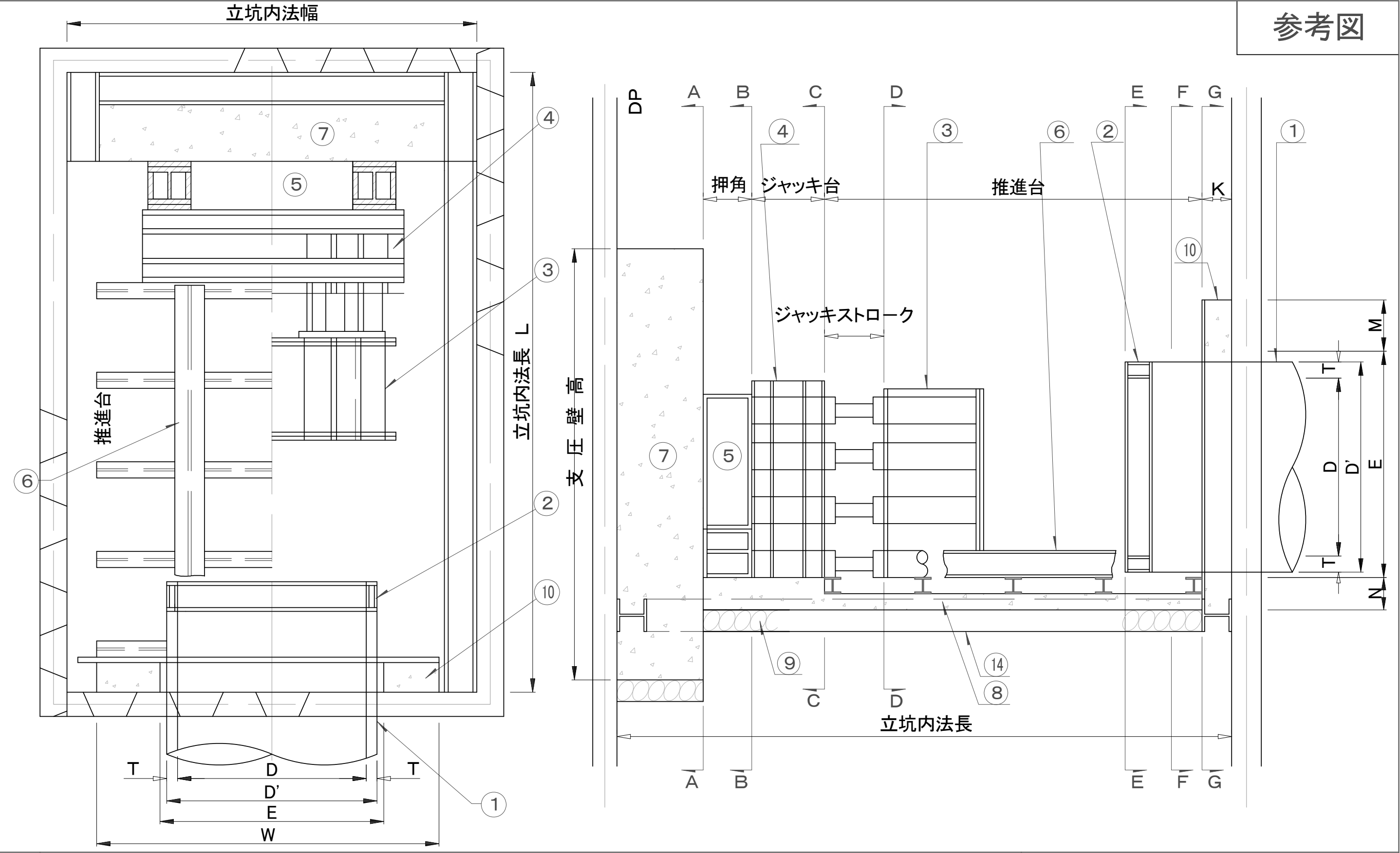
推進設備図(1)
