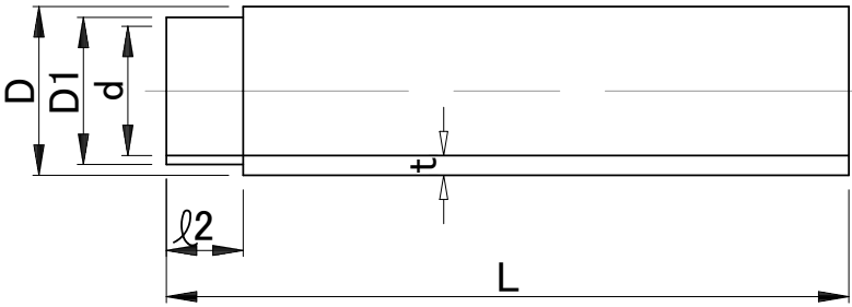
接続部参考図
