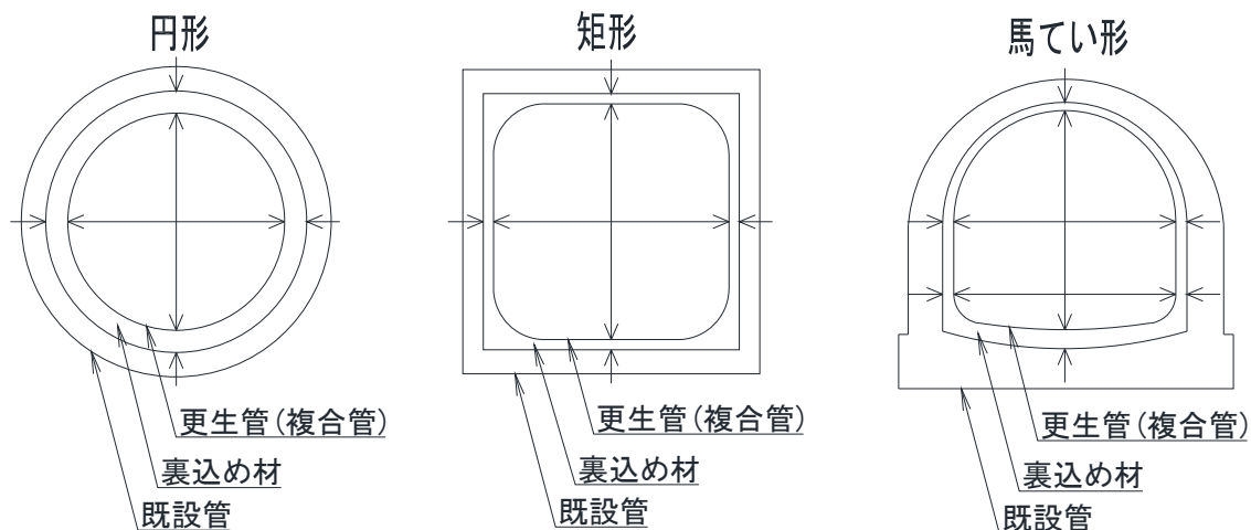
図 7-1 仕上り内径の測定位置
