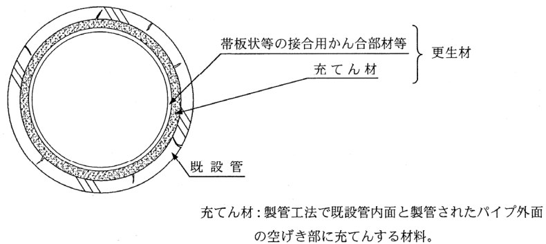
図10.4 複合管の概念
