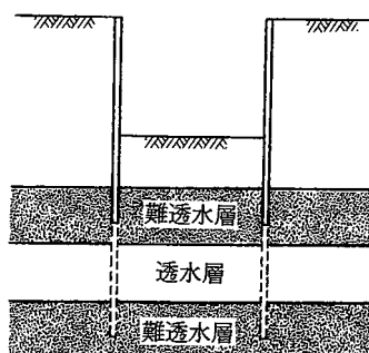
図8.12 根入れ長
