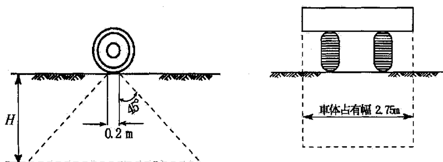
図3.23 活荷重の分布
