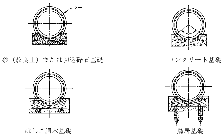
図3.8 剛性管きょの基礎工の種類
