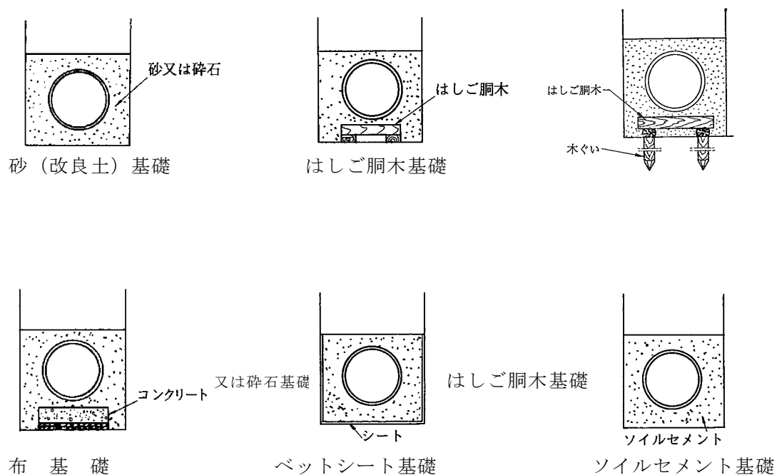
図3.9 可とう性管きょの基礎工の種類
