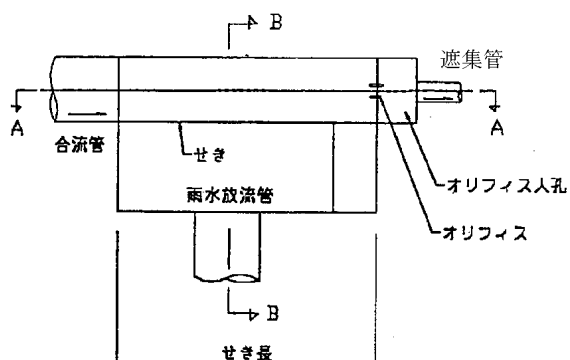
図5.5 完全横越流ぜき
