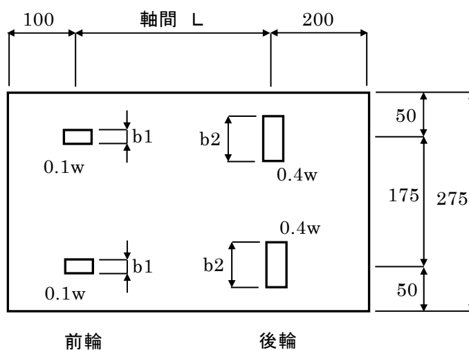
図8.3 T 荷重 (単位 : cm)
