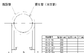
更生工断面図 (参考)
