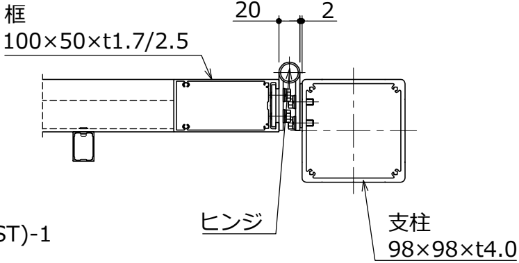
ヒンジ部 詳細図 S=1:5
