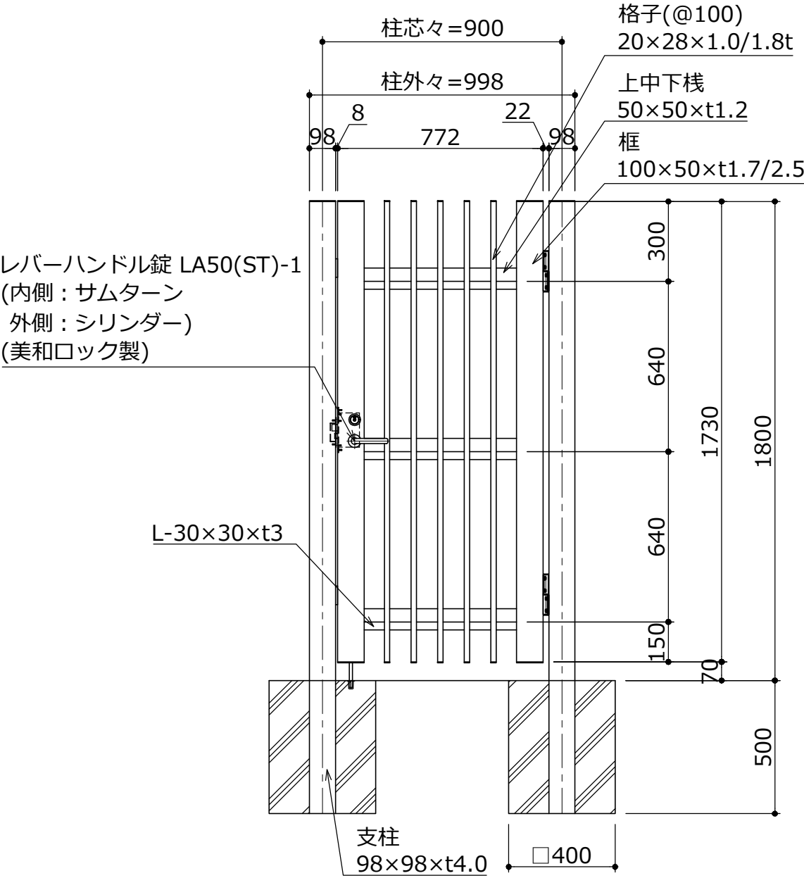
正面図 S=1:20
