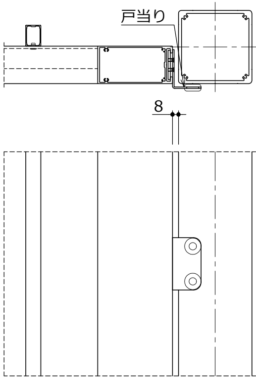
戸当り部(内観) 詳細図 S=1:5
