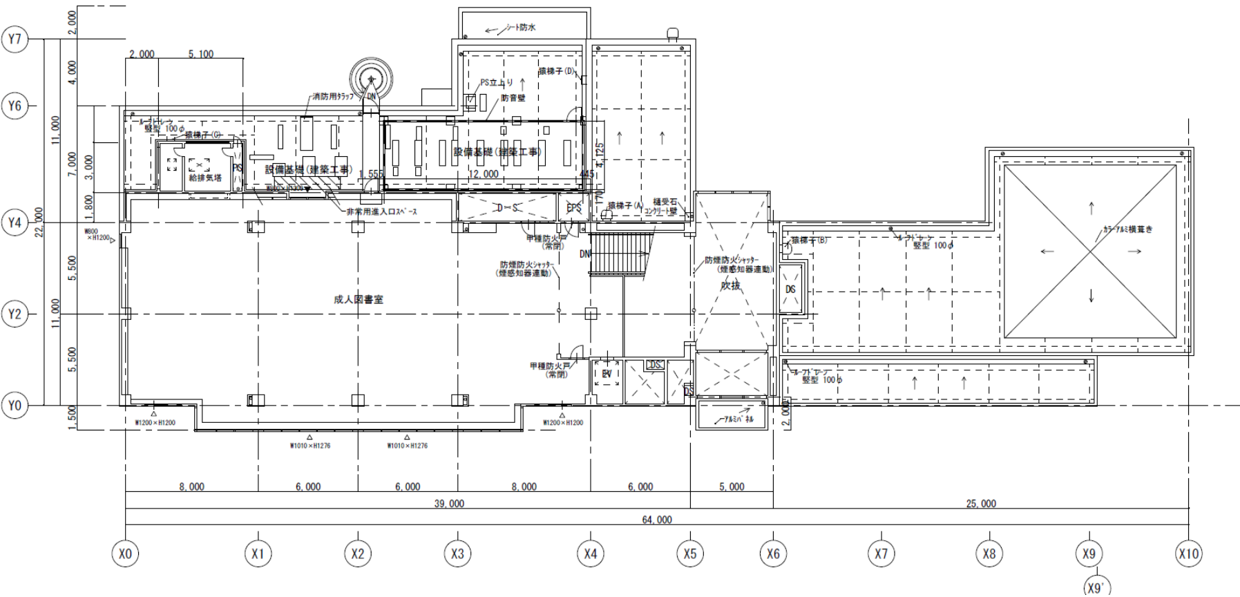
3階平面図
