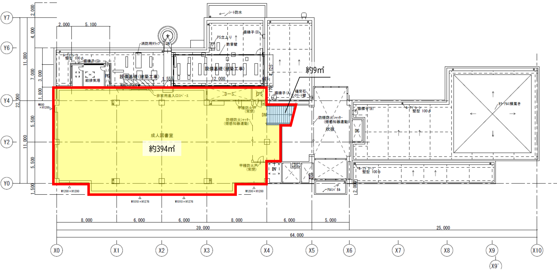
3階平面図
