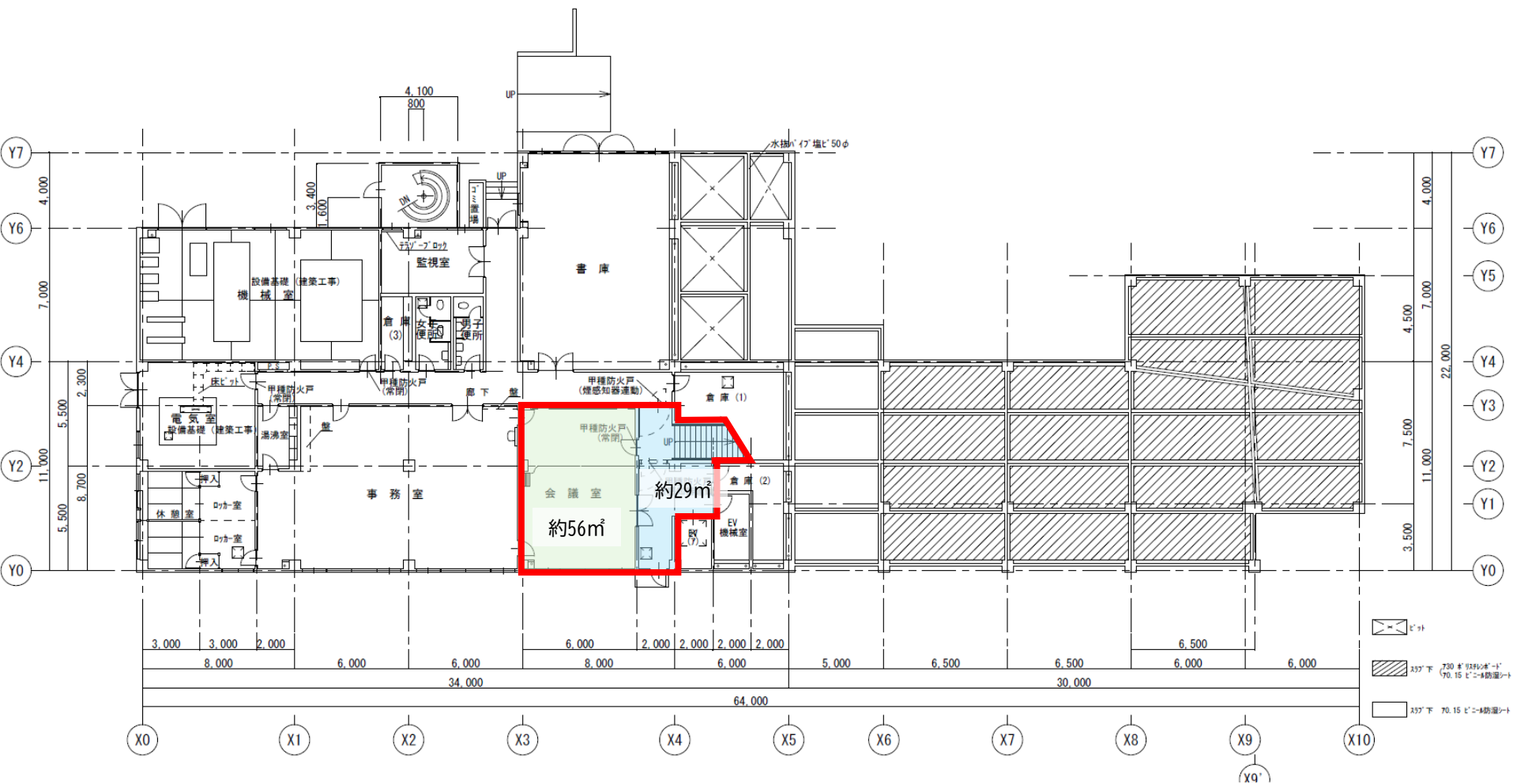
1階平面図
