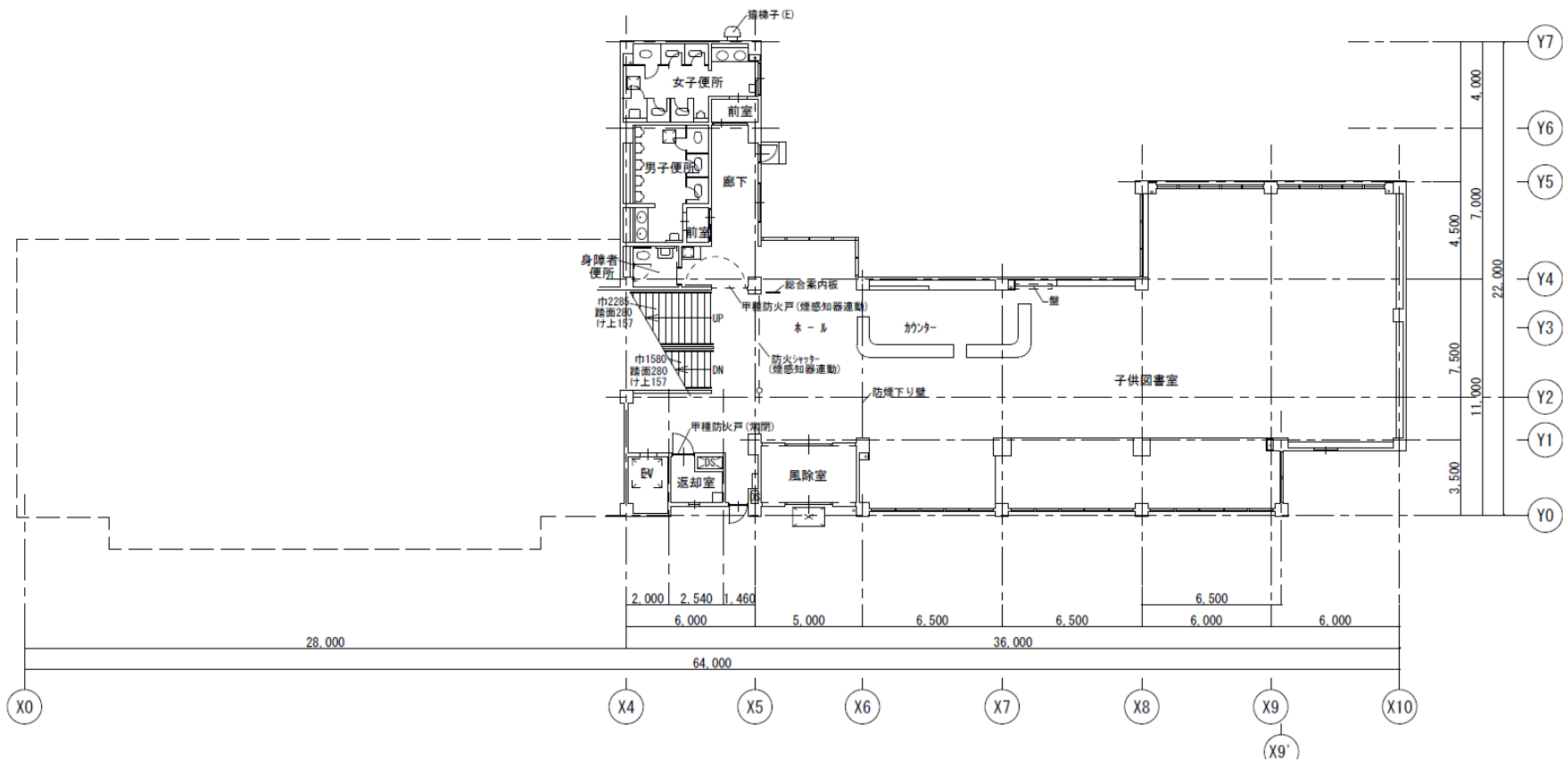
2階平面図
