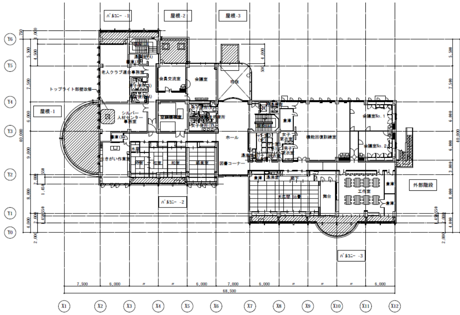
2階平面図
