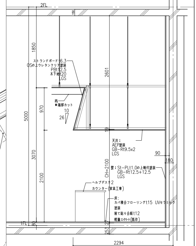
A断面図 S=1/50
