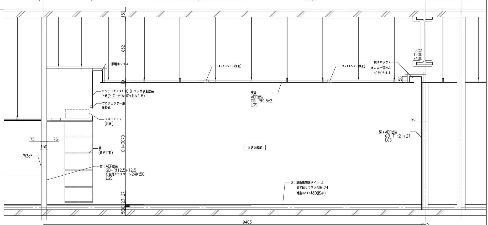
⑦5 C断面図 S=1/50
