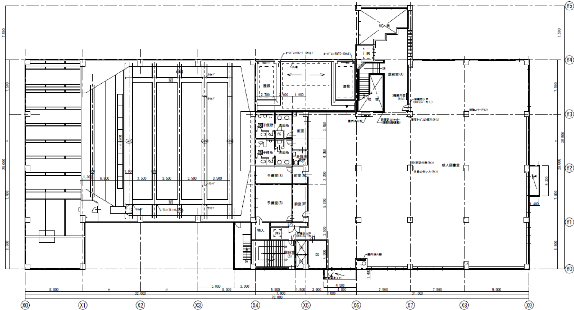
3階平面図
