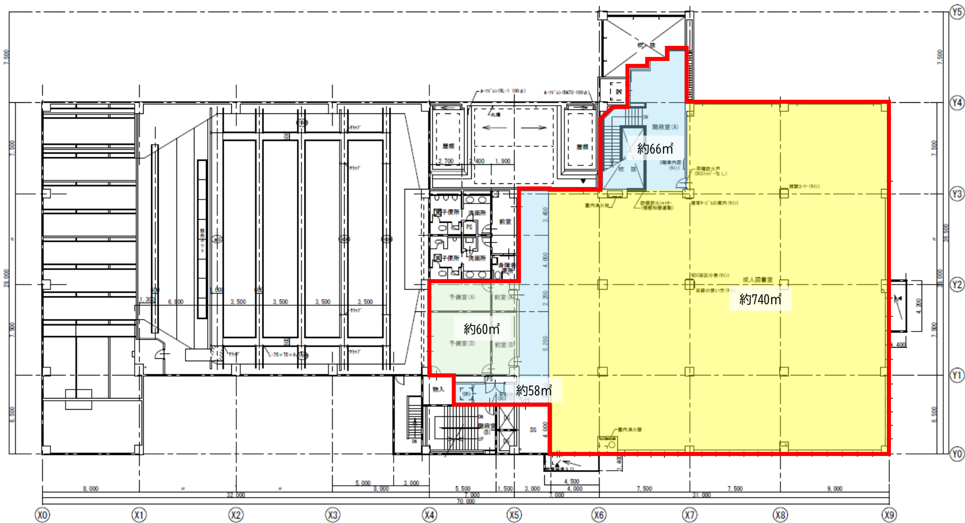
3階平面図
