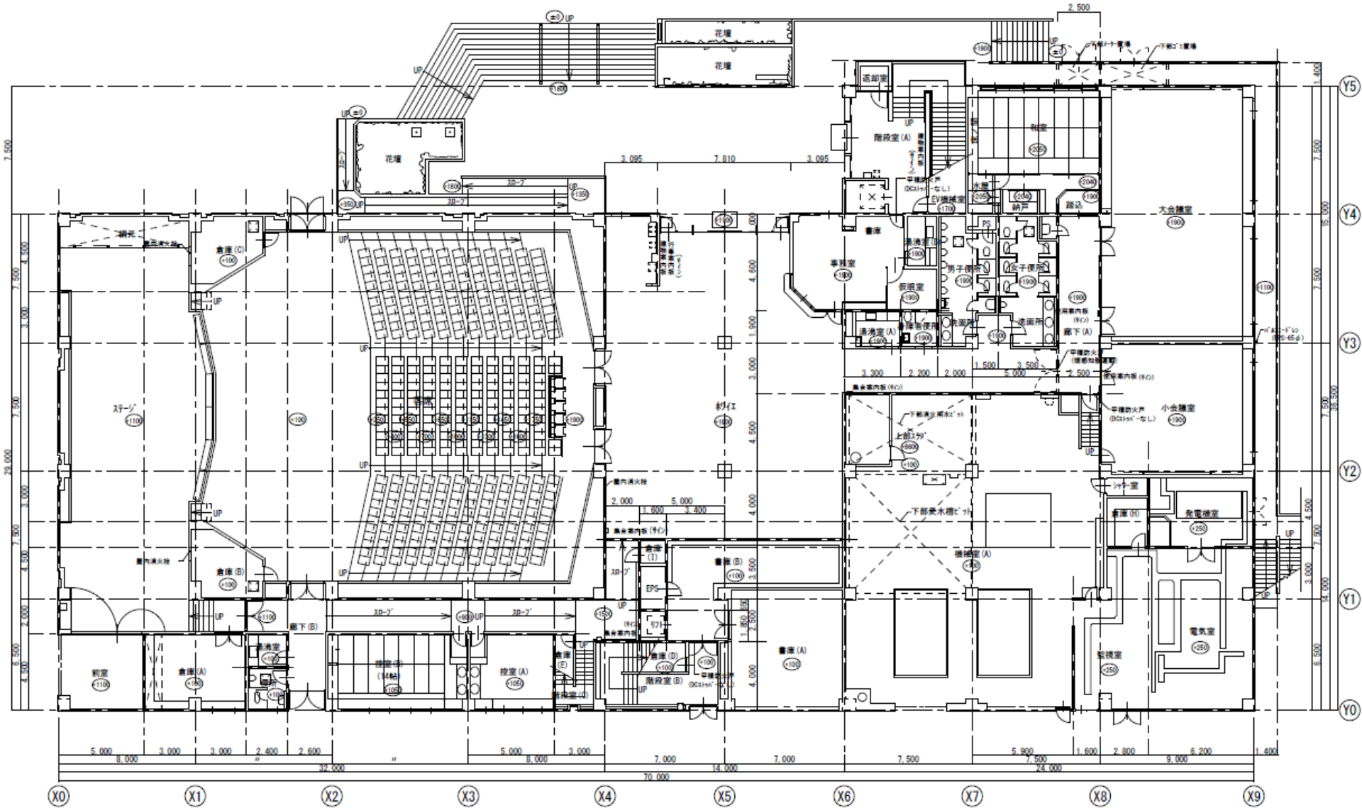
1階平面図
