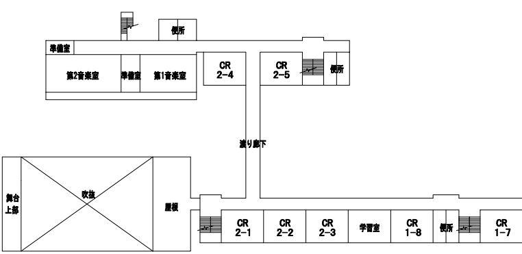
3階平面図
