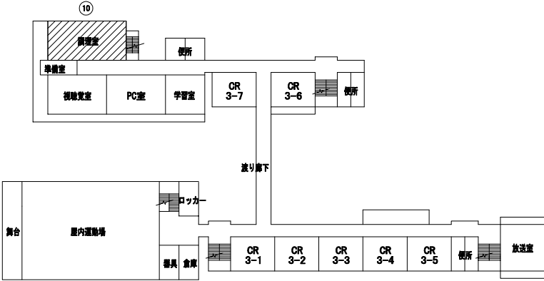
3階平面図
