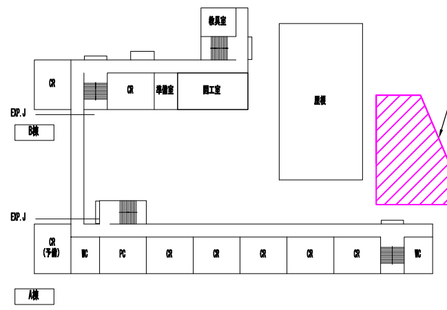
3階平面図
