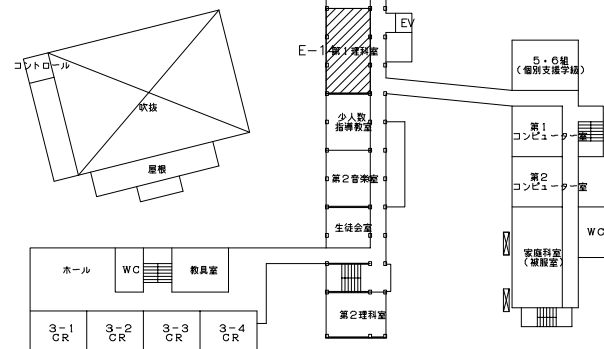
2階平面図
