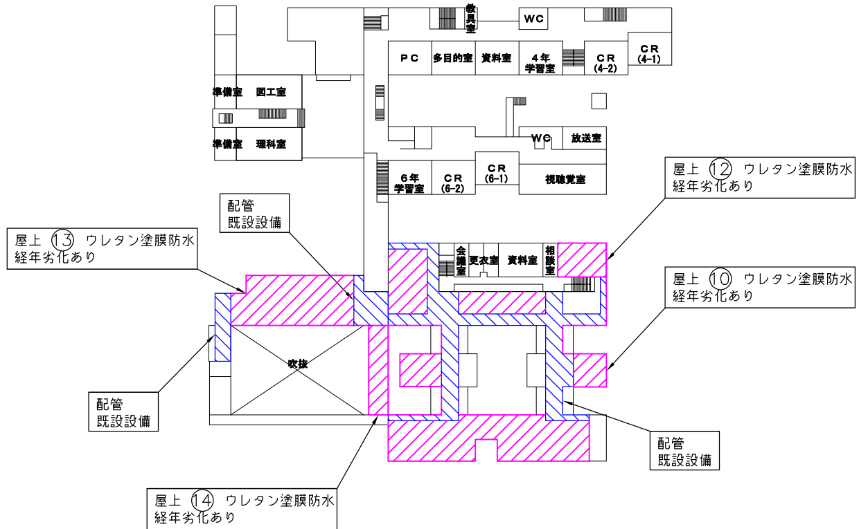
2階平面図
