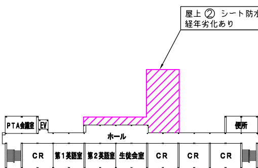
4階平面図
