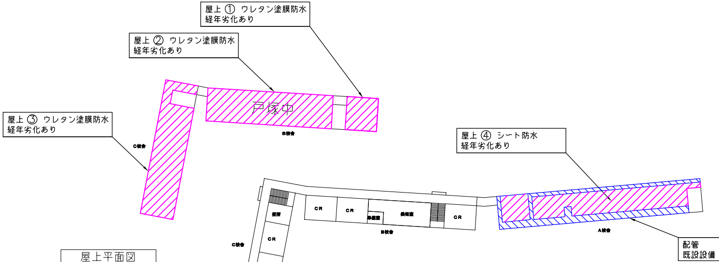
屋上平面図
