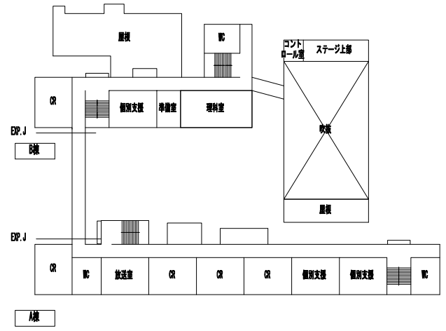
2階平面図
