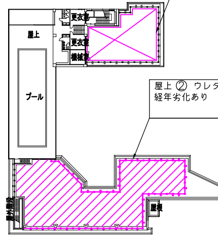
4階平面図
