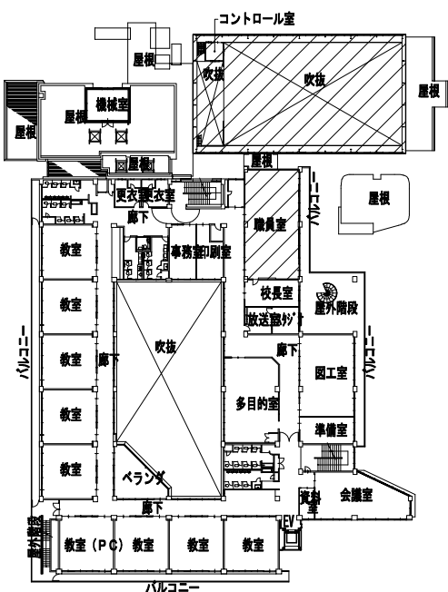
2階平面図
