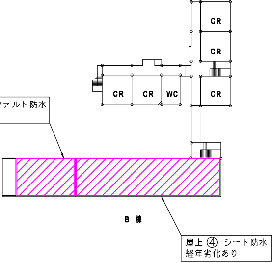
4階平面図
