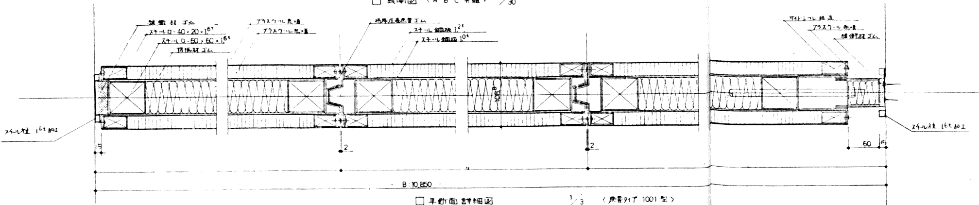
□ 断面図 1/30 (標準型 1001 型)
