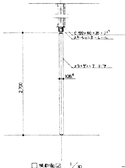
□ 断面図 1/30
