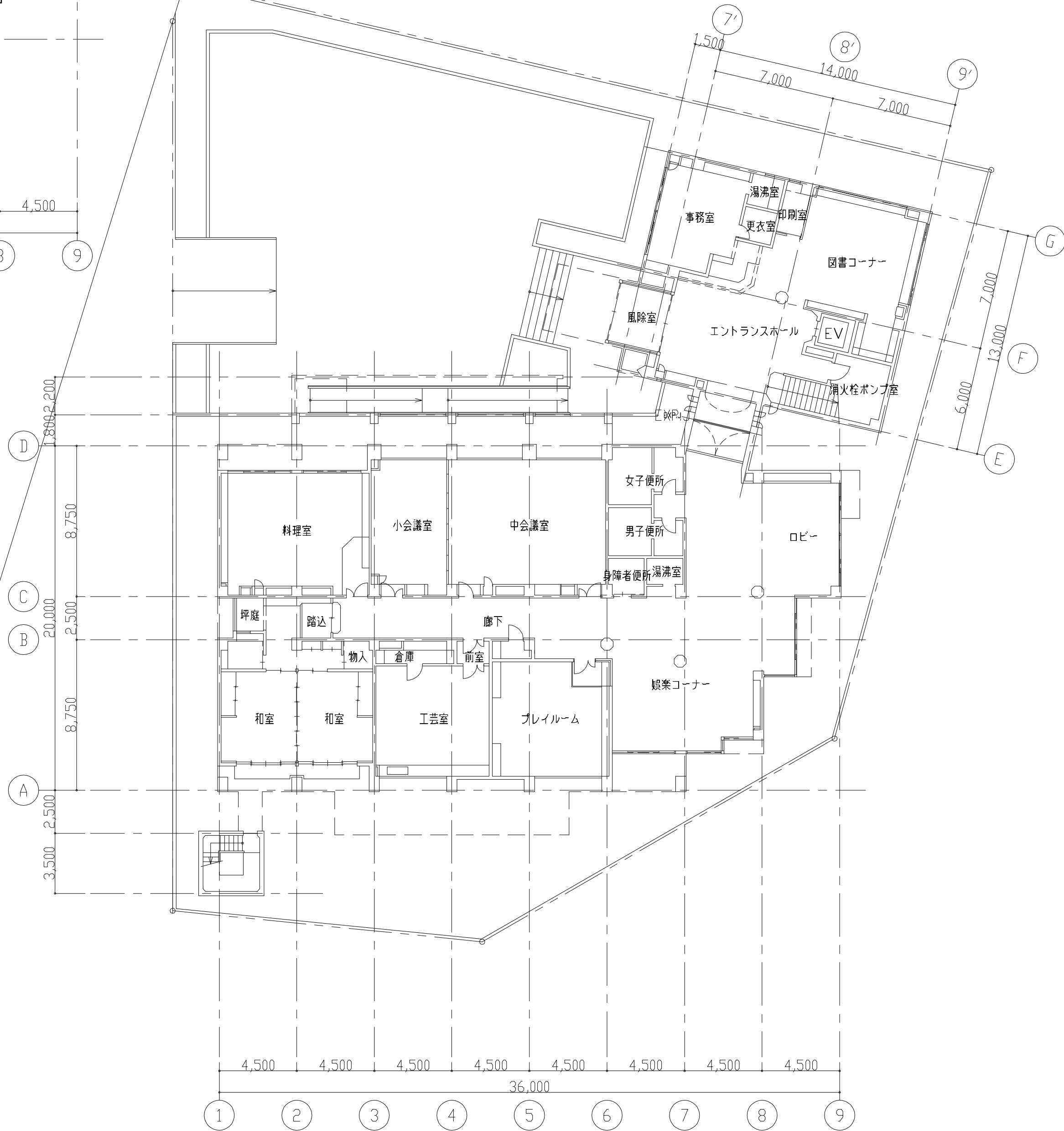
配置図・1階平面図 1:200
