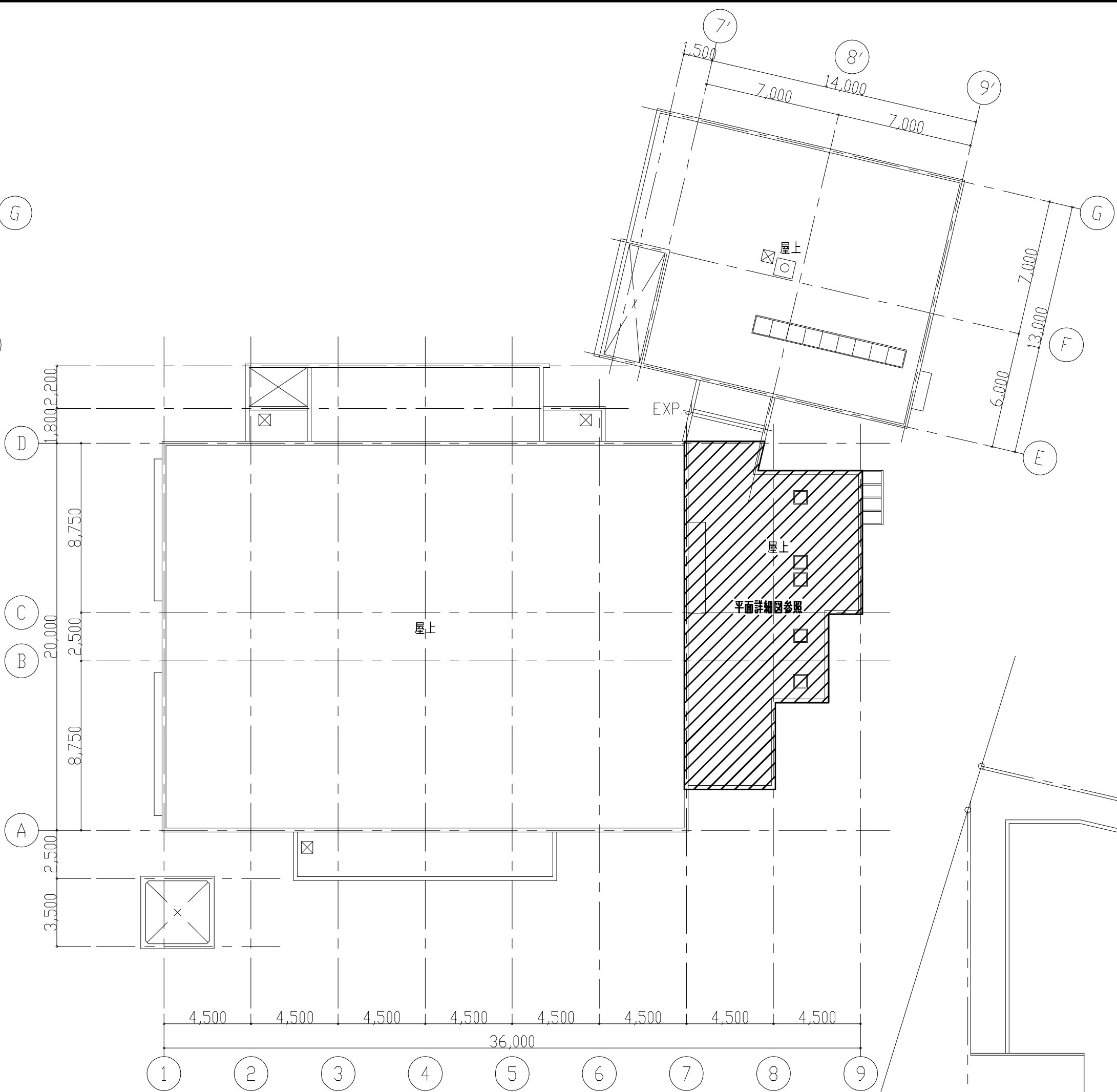
R階平面図 1:200
