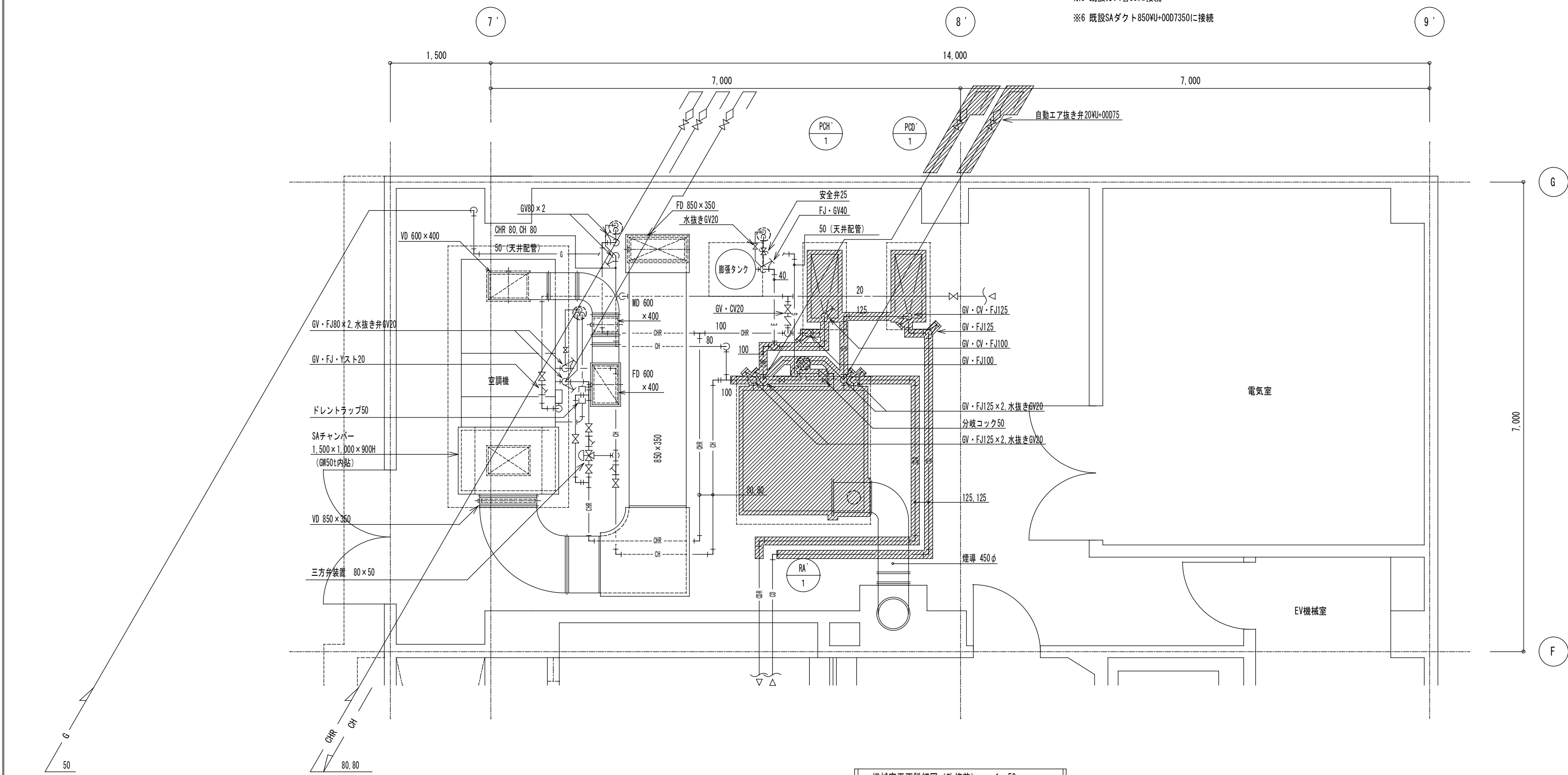
機械室平面詳細図 (改修前) 1 : 50
