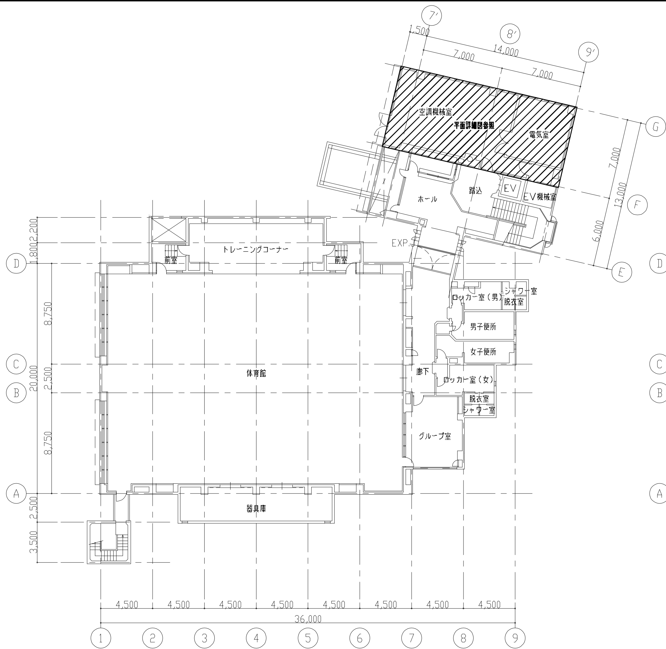
2階平面図 1:200
