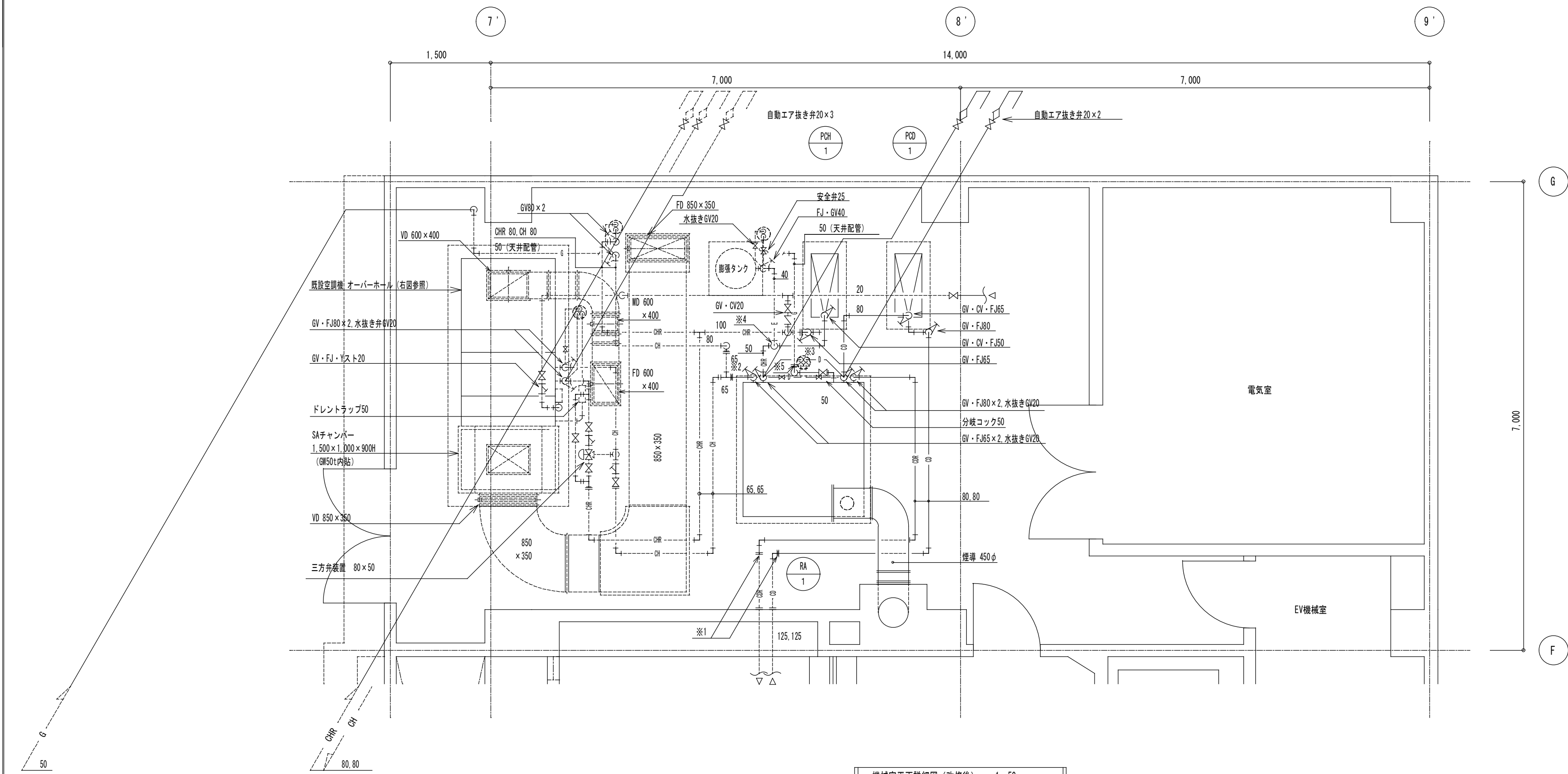
機械室平面詳細図 (改修後) 1 : 50
