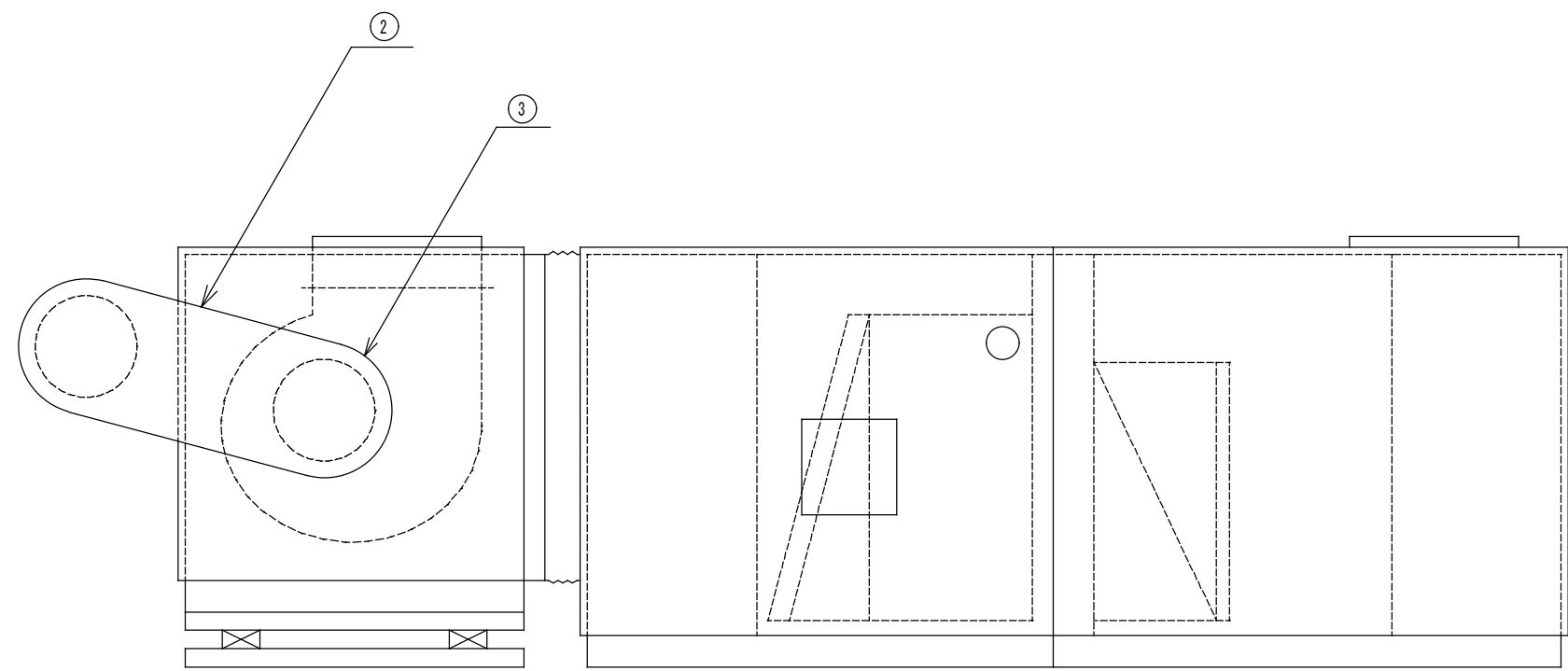
立面姿図
