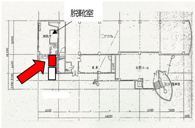
脱靴室 エレベーター エレベーターホール 2200 2350 4650 5000 5500 4650 5500 7500 2500
