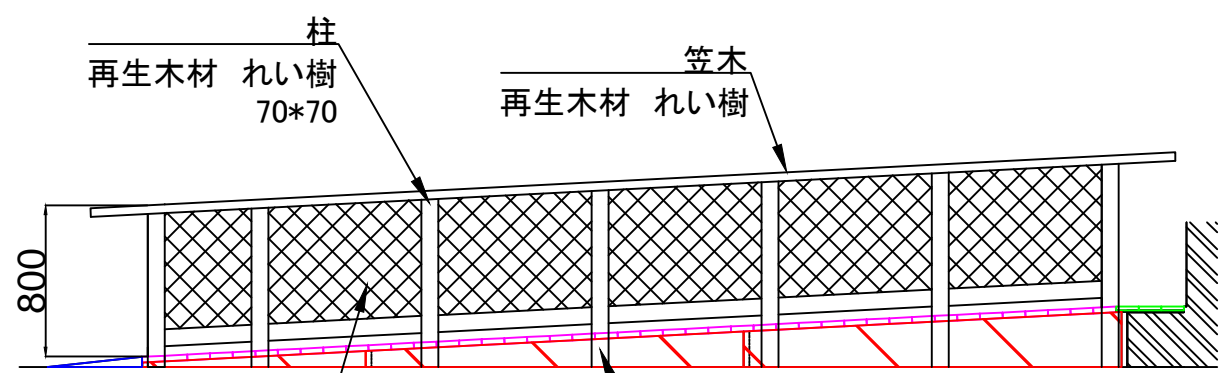
B-B断面図
