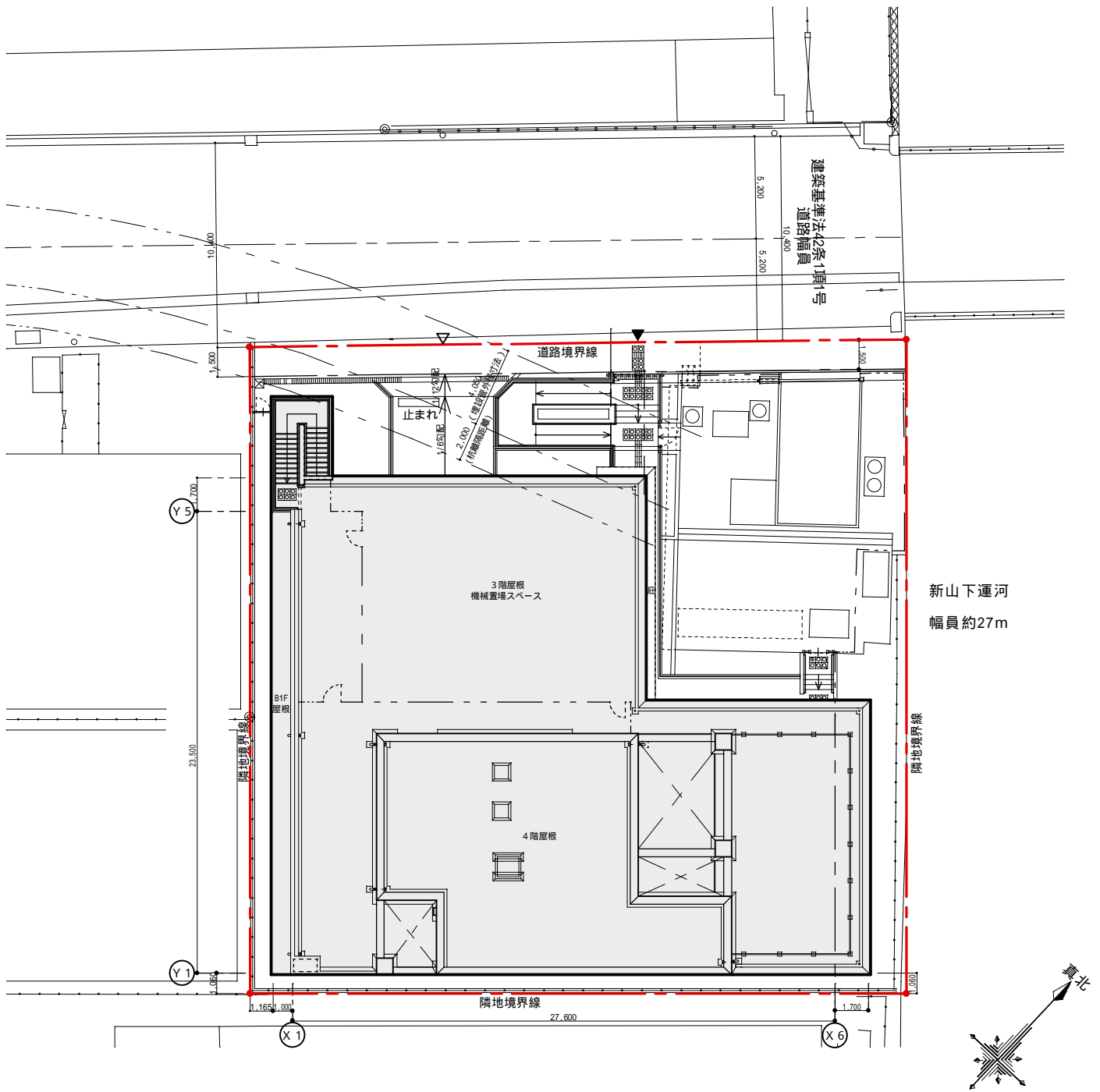
配置図 1/300
