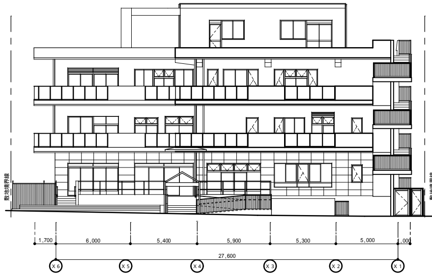
北側立面図 1/300
