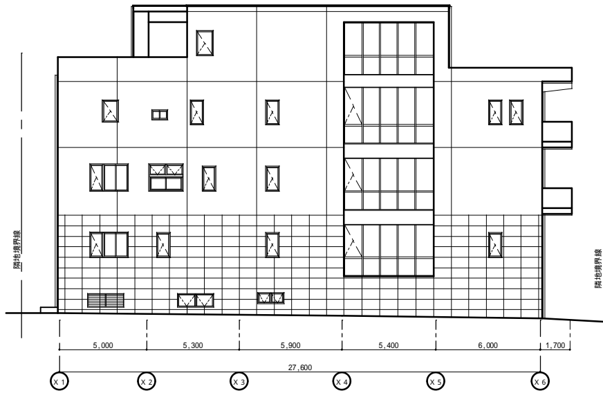
南側立面図 1/300
