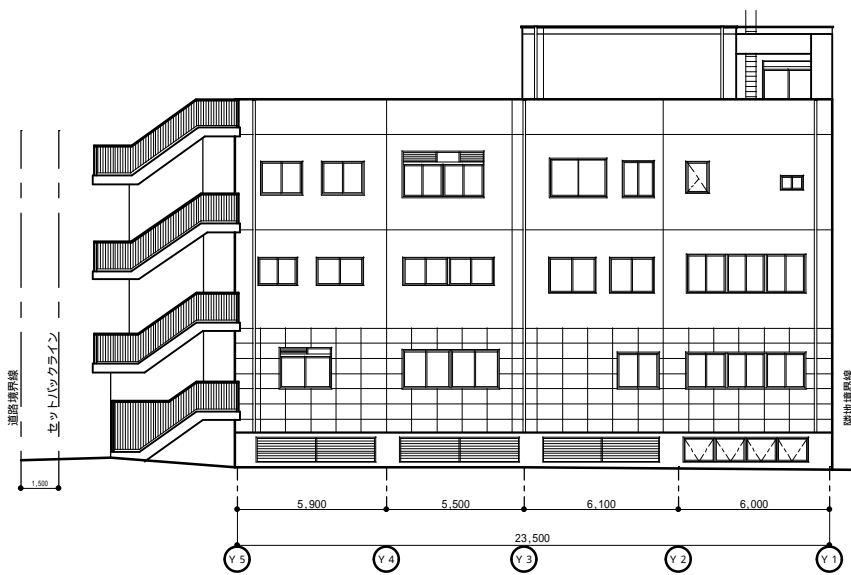
西側立面図 1/300
